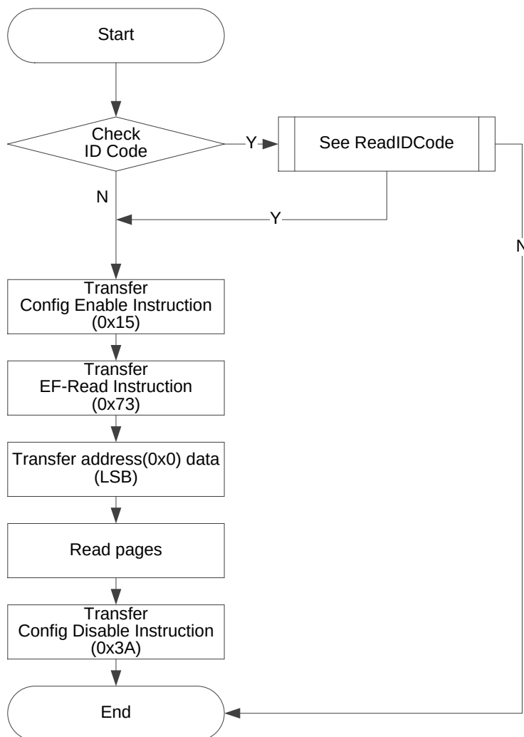
图 7-22 读取内部 Flash 流程图
