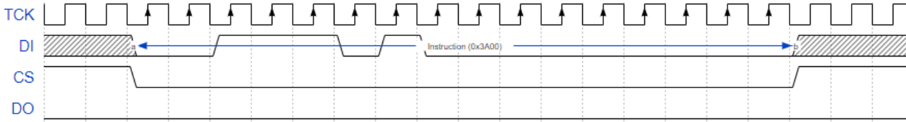
图 7-39 Write Disable (0x3A00) 时序示意图
