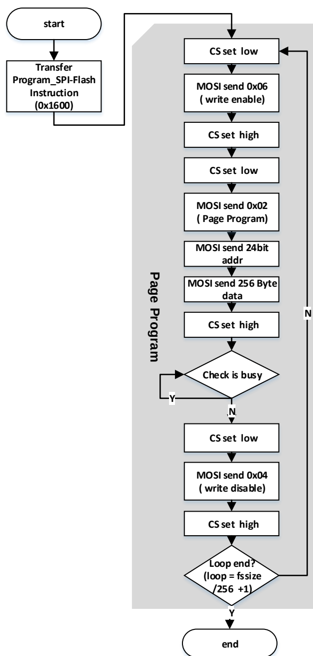
图 7-46 SPI-Flash 编程一个 page 流程图
