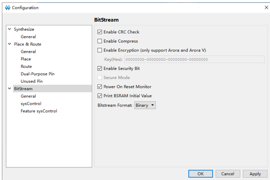
图 3-1 配置选项
