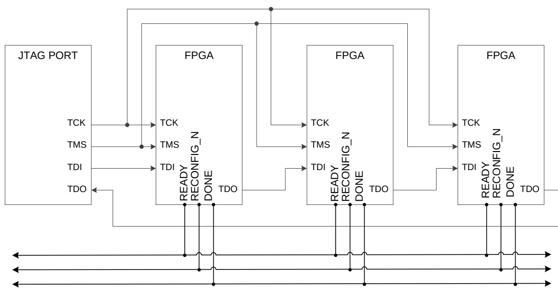
图 7-5 JTAG 菊花链配置模式连接示意图
