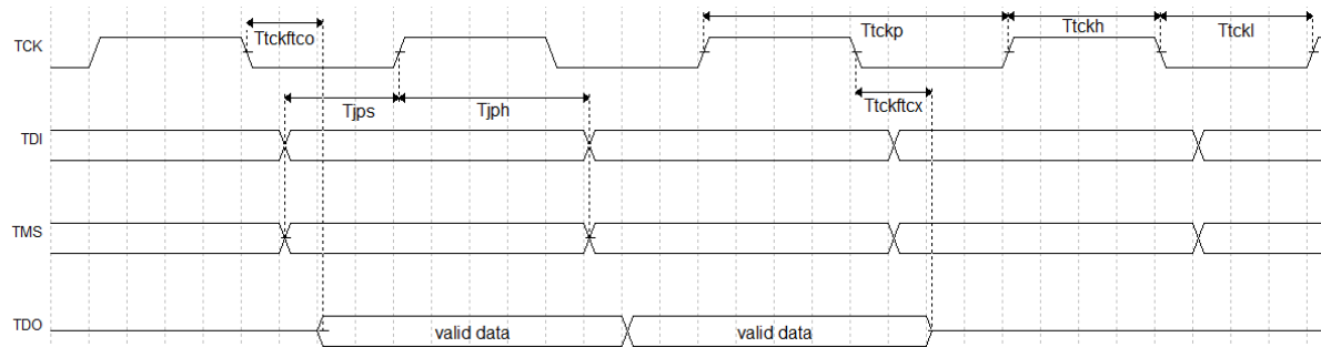
图 7-6 JTAG 配置模式时序图
