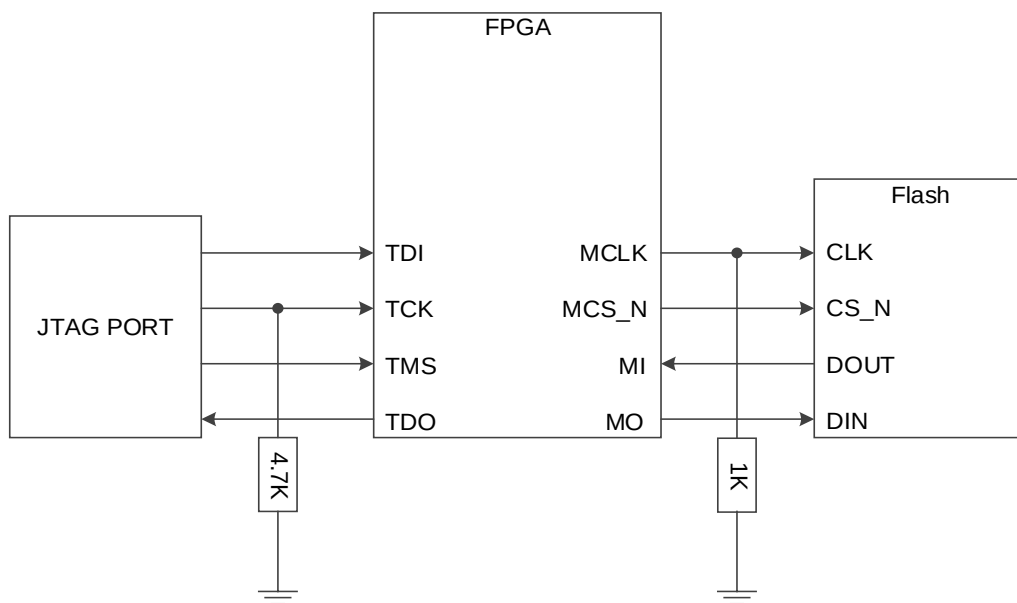
图 7-26 JTAG 接口编程外部 Flash 连接示意图(GW2A(R)-18/GW2A-55/小蜜蜂家族)
