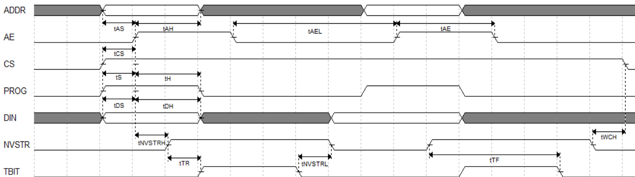
图 3-16 FLASH128K 写操作模式
