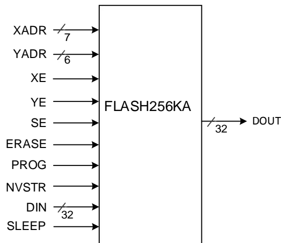
图 3-23 FLASH256KA 端口示意图
