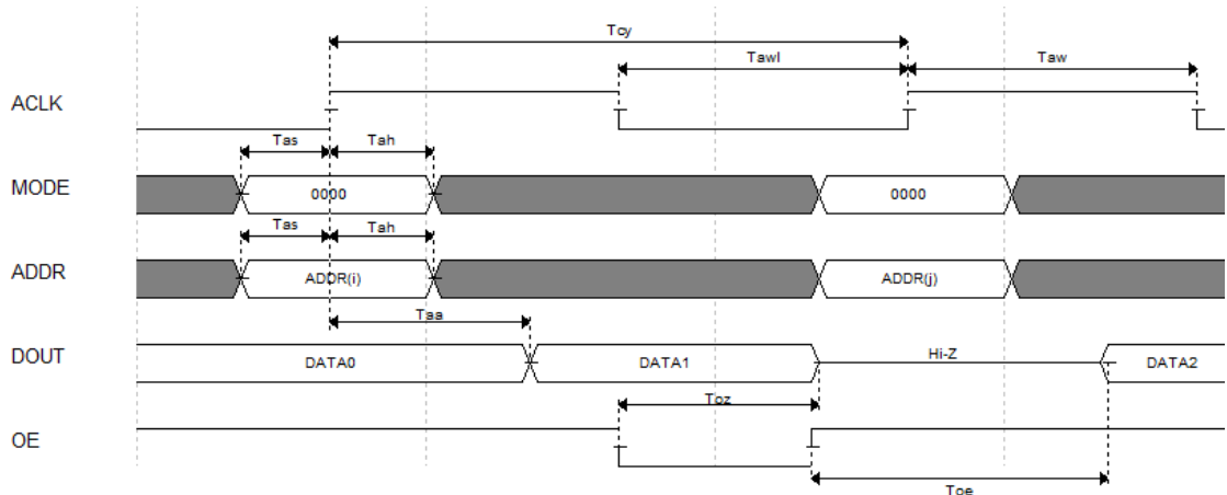
图 3-2 FLASH96K 读操作模式
