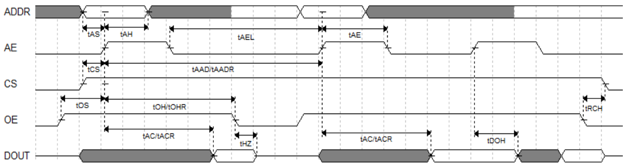
图 3-15 FLASH128K 读操作模式
