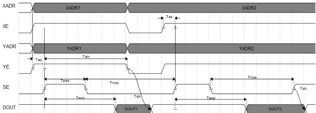
图 3-25 FLASH608K 读操作时序
