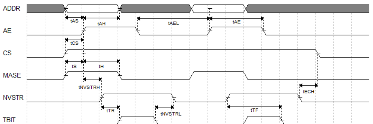
图 3-18 FLASH128K 模块擦除模式
