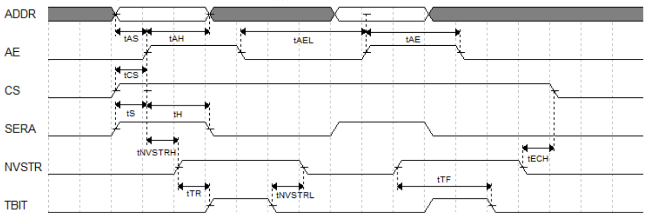
图 3-17 FLASH128K 页擦除模式
