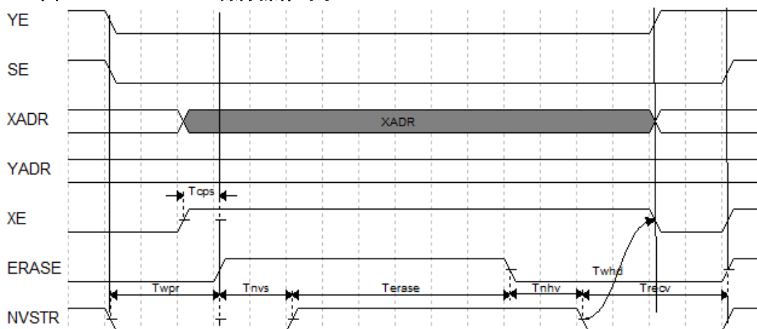
图 3-22 FLASH256K 擦除操作时序
