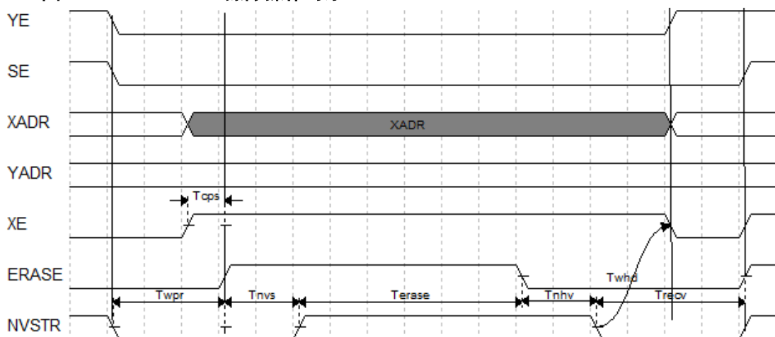
图 3-17 FLASH256K 擦除操作时序
