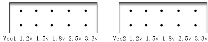
图 2-11 vcc1 vcc2 配置接口示意图
