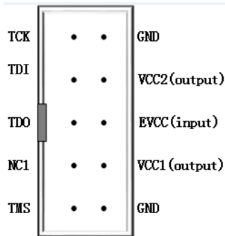
图 2-10 烧录接口连线示意图
