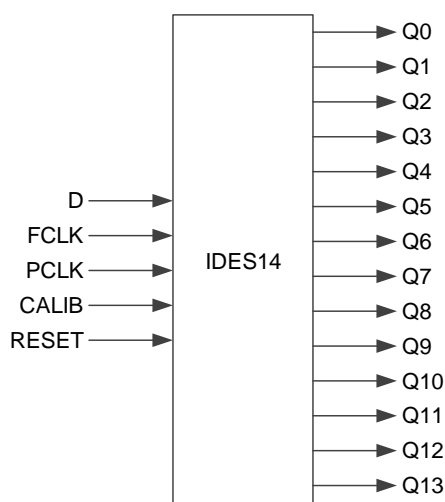
图 4-22 IDES14 端口示意图
