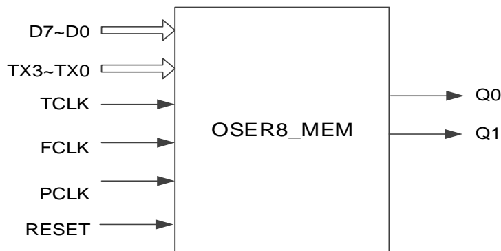
图 4-42 OSER8_MEM 端口示意图
