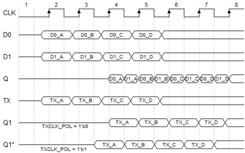
图 4-26 ODDR 时序图
