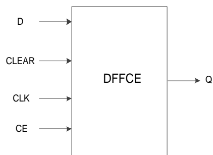
图 4-6 DFFCE 端口示意图
