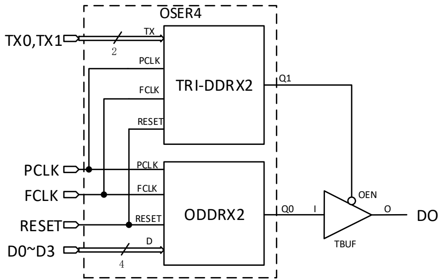
图 4-30 OSER4 逻辑框图
