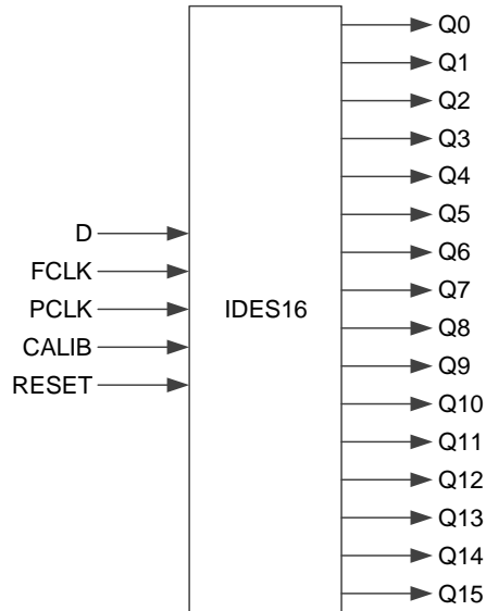
图 4-18 IDES16 端口示意图
