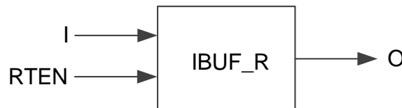
图 3-16 IBUF_R 端口示意图
