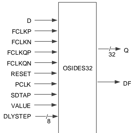
图 4-24 OSIDES32 端口示意图
