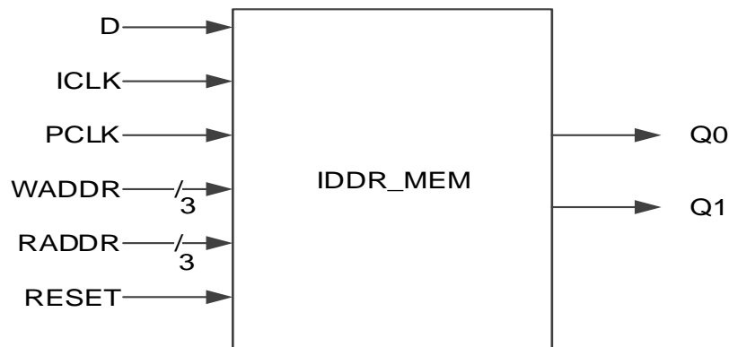
图 4-19 IDDR_MEM 端口示意图
