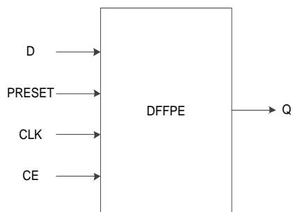
图 4-5 DFFPE 端口示意图
