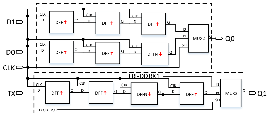
图 4-25 ODDR 逻辑框图
