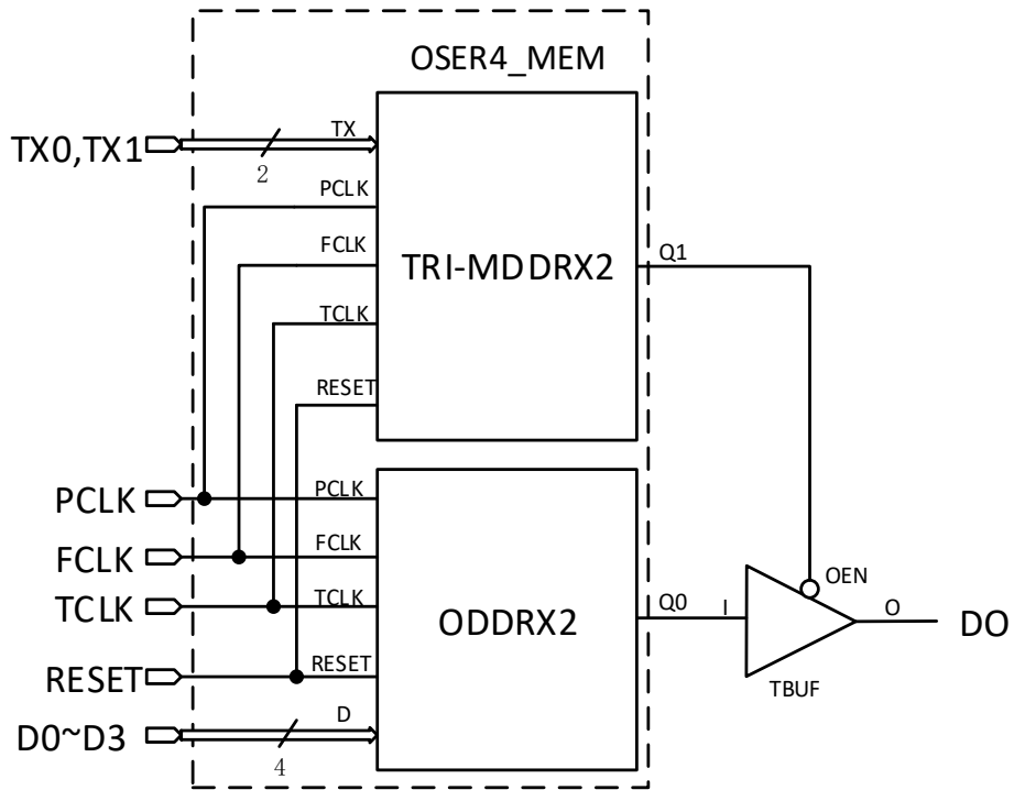
图 4-39 OSER4_MEM 逻辑框图
