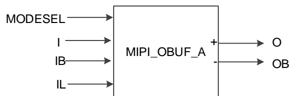
图 3-14 MIPI_OBUF_A 端口示意图
