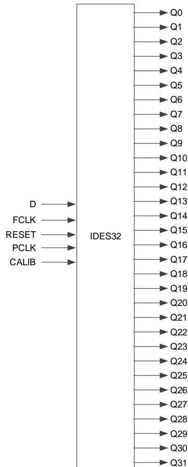
图 4-23 IDES32 端口示意图
