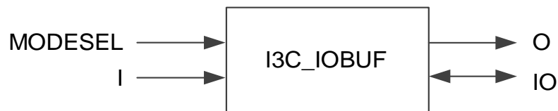
图 3-15 I3C_IOBUF 端口示意图
