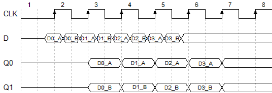
图 4-10 IDDR 时序图
