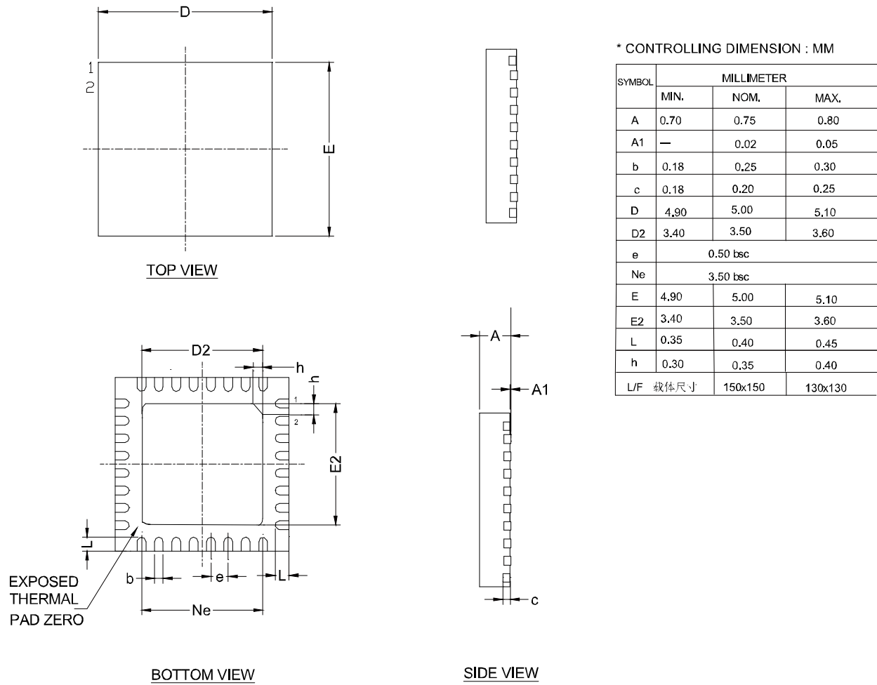
图 4-2 封装尺寸 QN32U
