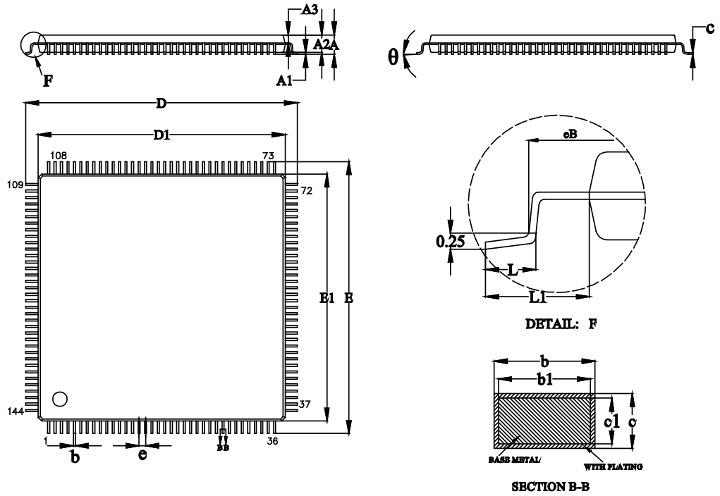
图 4-6 封装尺寸 LQ144
