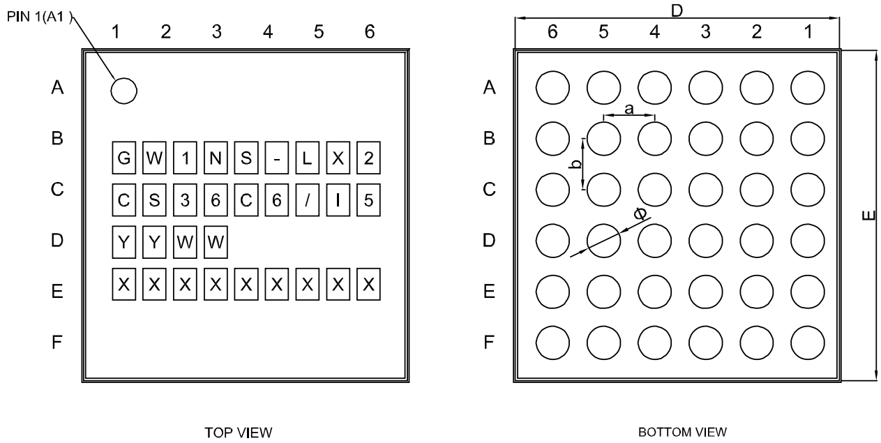
图 4-3 封装尺寸 CS36
