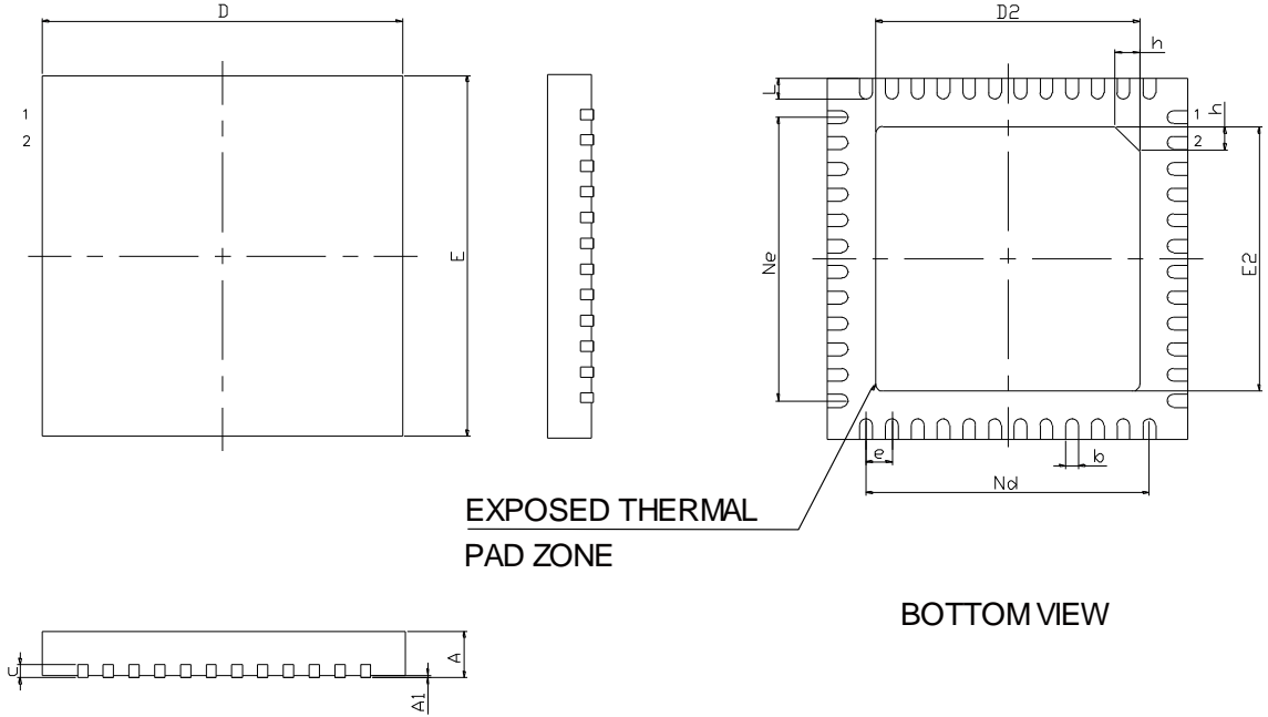
图 4-5 封装尺寸 QN48(GW1NS-4/GW1NS-4C)
