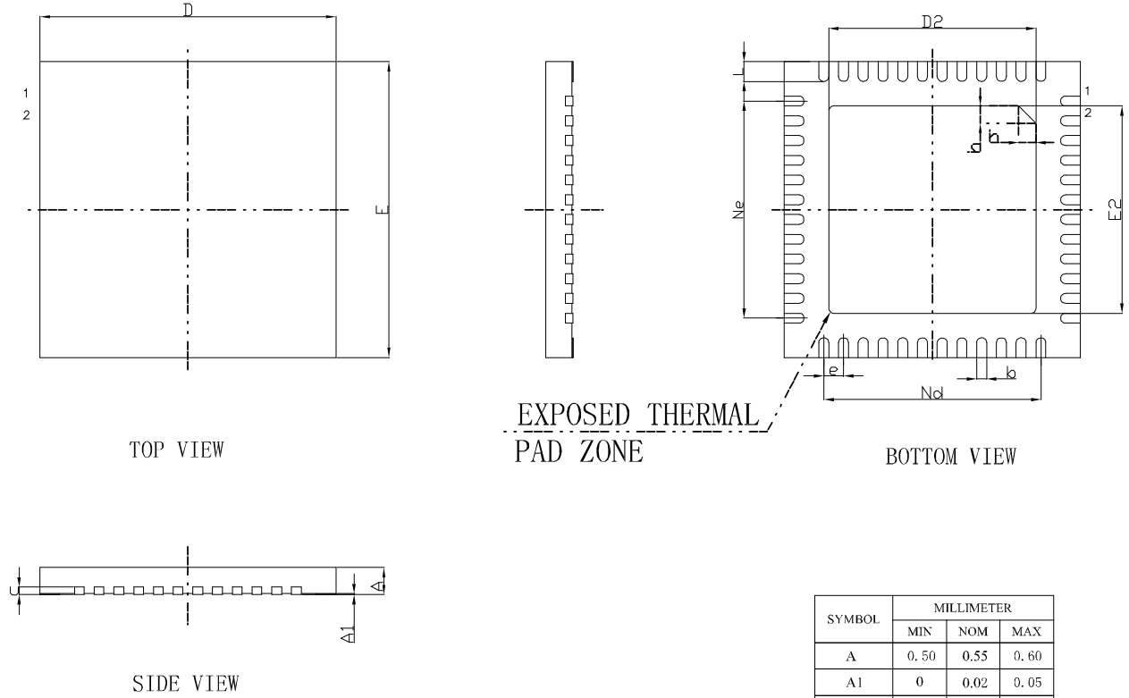
图 4-4 封装尺寸 QN48(GW1NS-2/GW1NS-2C)
