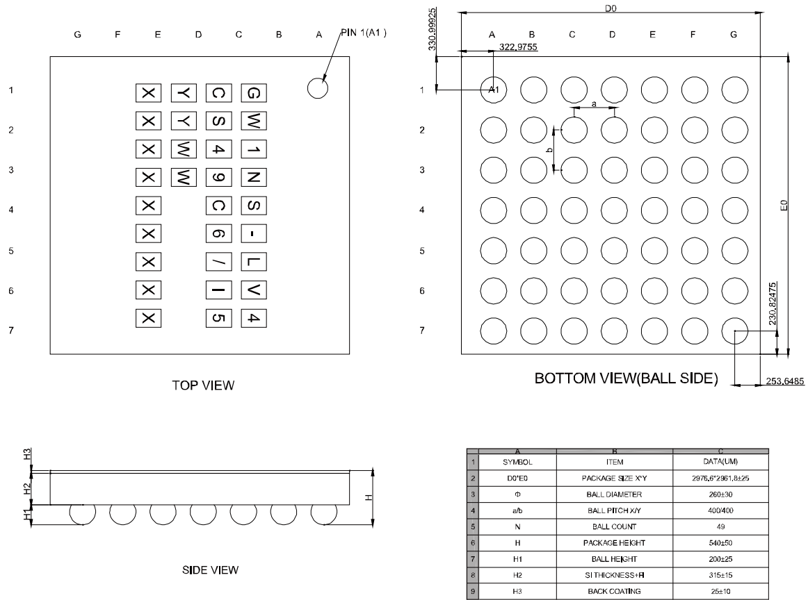
图 4-4 封装尺寸 CS49
