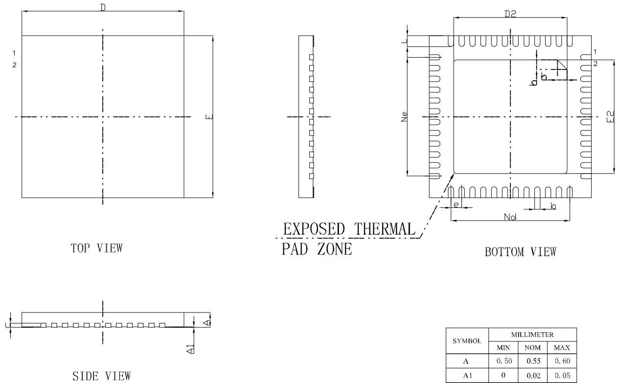
图 4-5 封装尺寸 QN48(GW1NS-2/GW1NS-2C)
