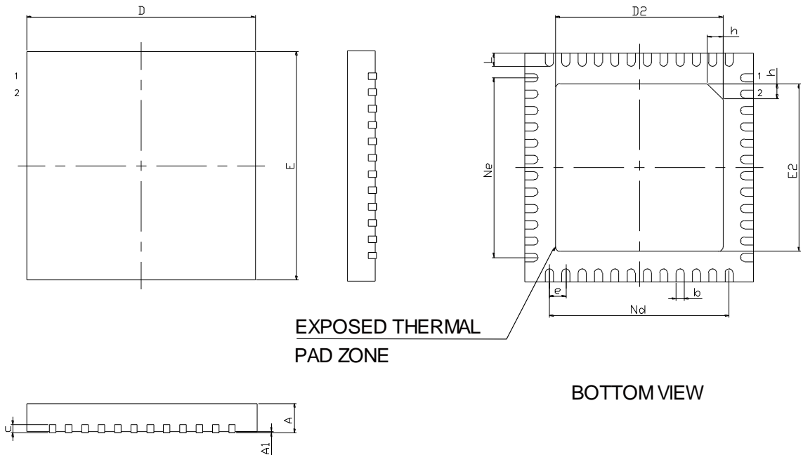
图 4-6 封装尺寸 QN48(GW1NS-4/GW1NS-4C)
