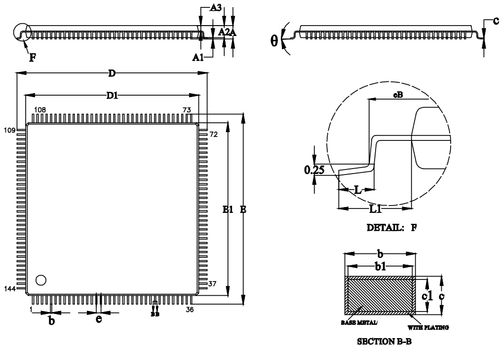
图 4-7 封装尺寸 LQ144
