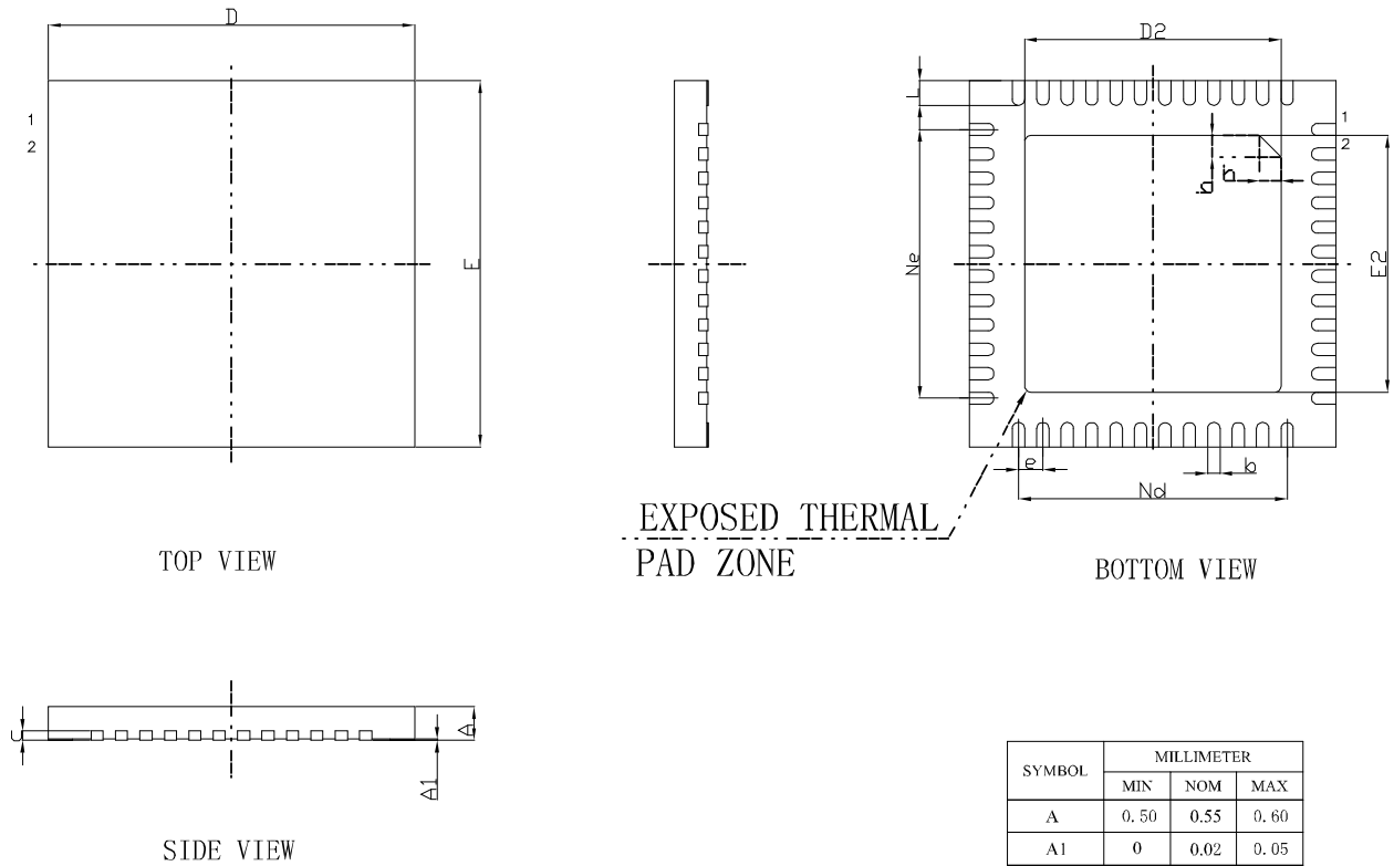
图 4-6 封装尺寸 QN48(GW1NS-2/GW1NS-2C)
