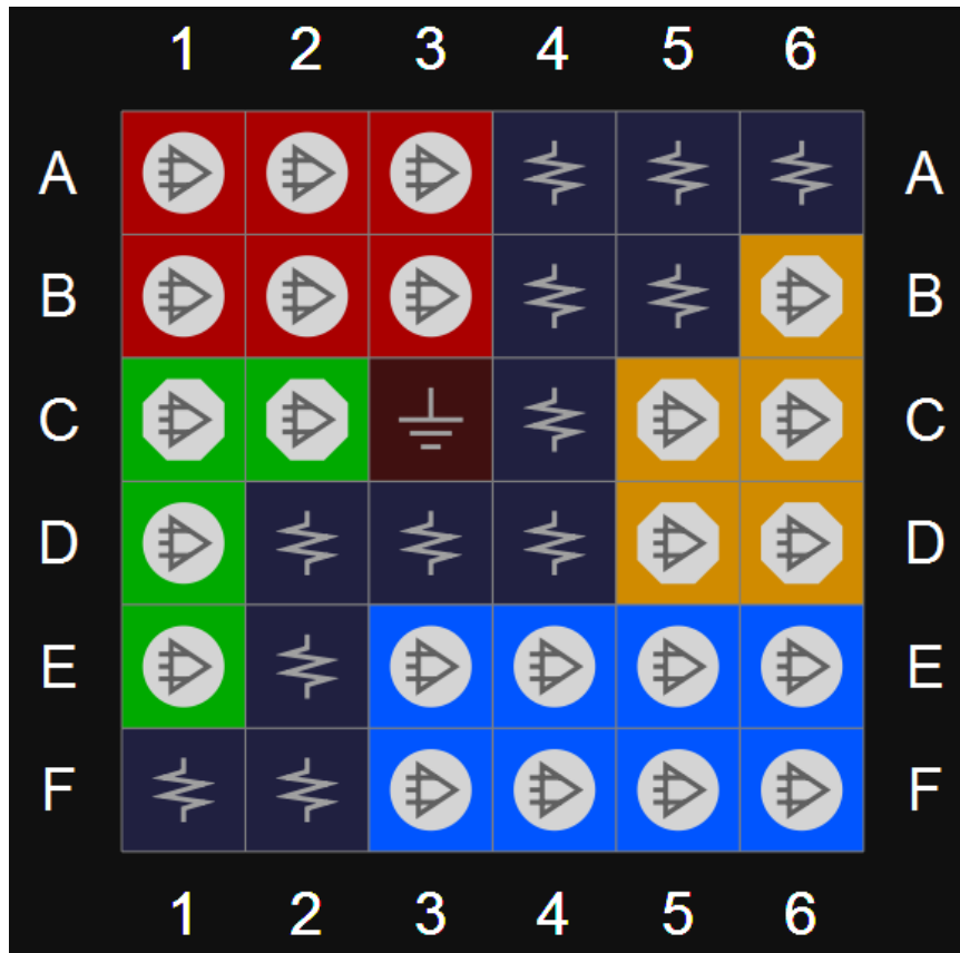
GW1NS-2/GW1NS-2C 器件 CS36U 其他管脚
