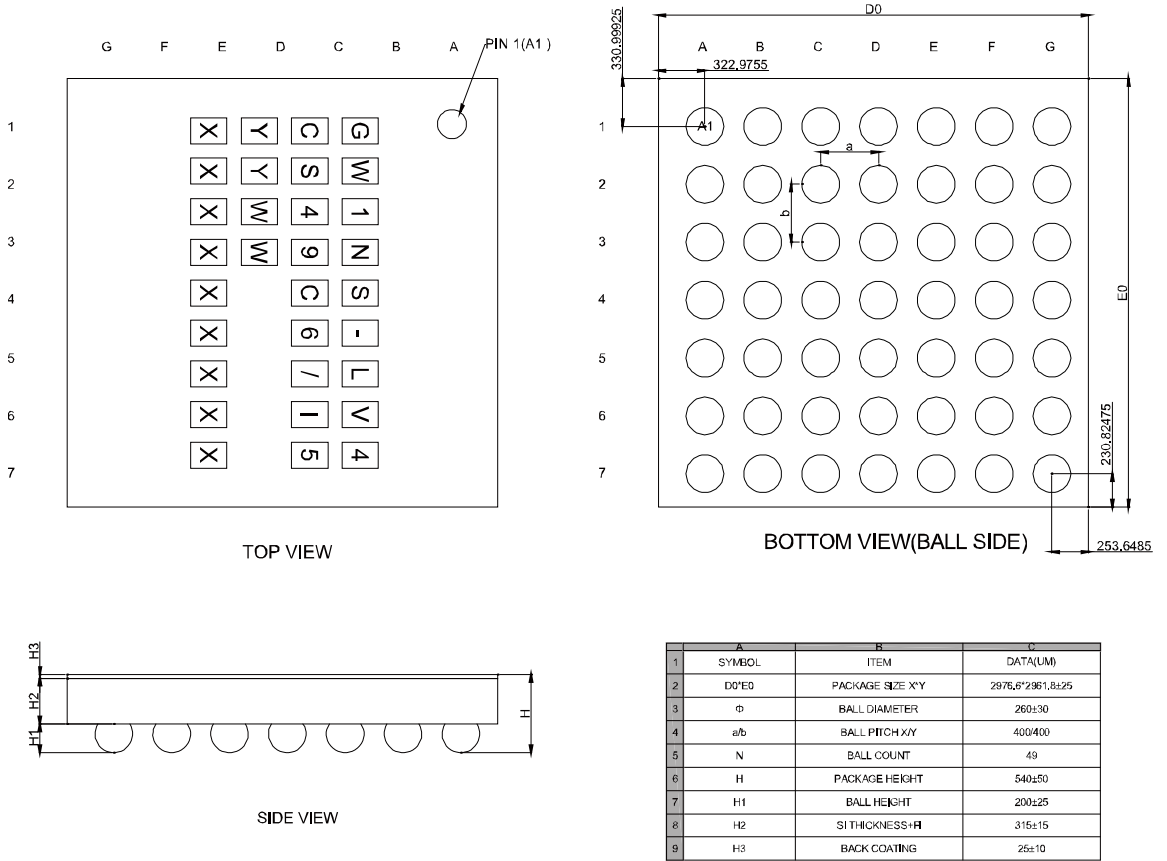
图 4-5 封装尺寸 CS49
