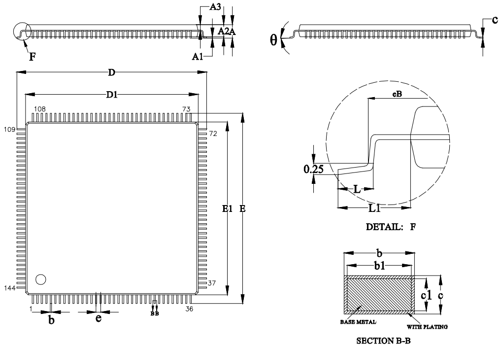
图 4-8 封装尺寸 LQ144
