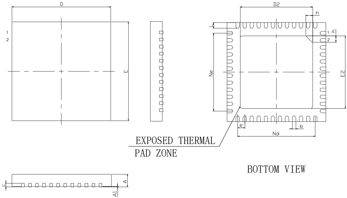
图 4-6 封装尺寸 QN48(GW1NS-2/GW1NS-2C)
