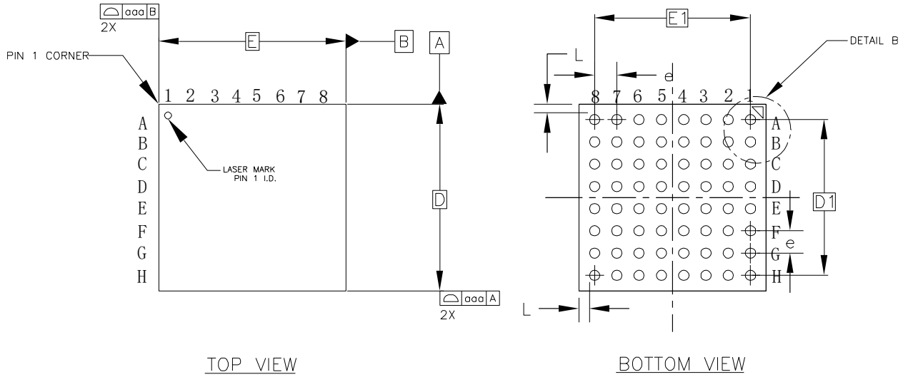
图 4-9 封装尺寸 MG64
