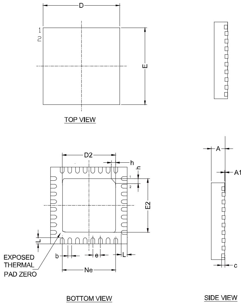
图 4-1 封装尺寸 QN32
