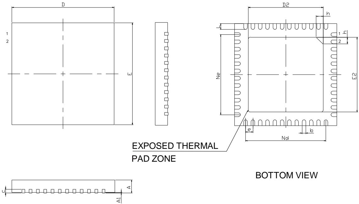
图 4-7 封装尺寸 QN48(GW1NS-4/GW1NS-4C)
