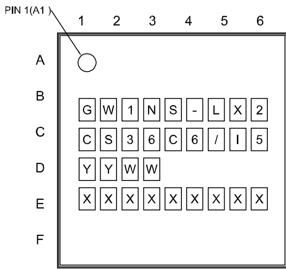
图 4-3 封装尺寸 CS36
