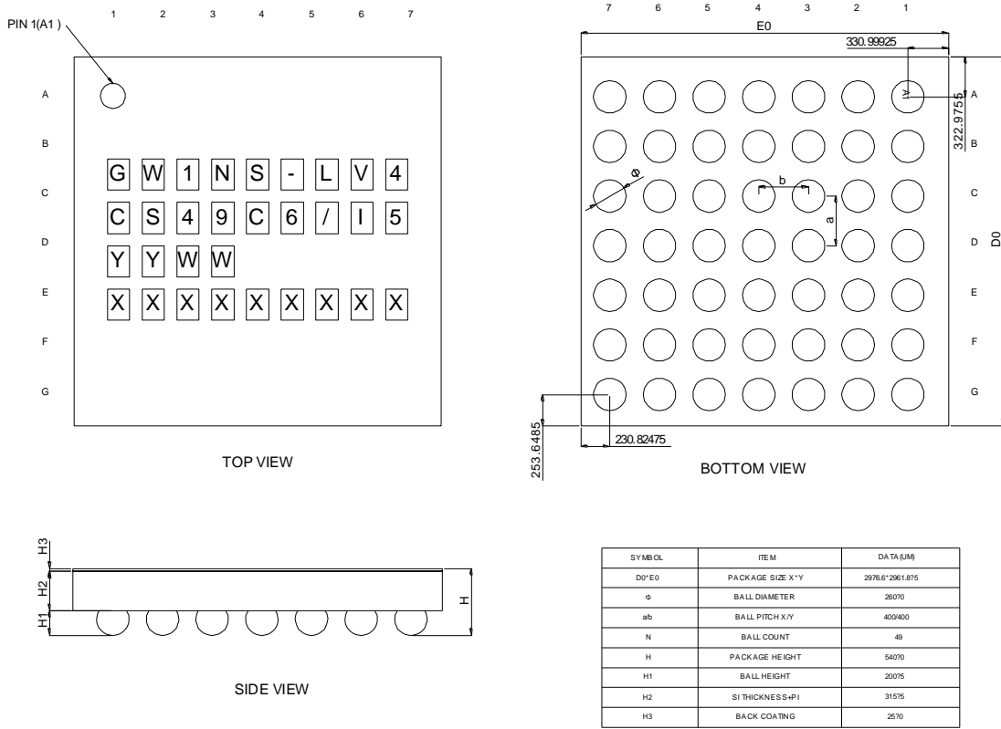
图 4-5 封装尺寸 CS49
