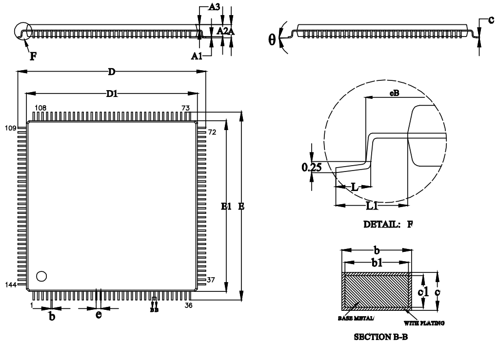
图 4-7 封装尺寸 LQ144X
