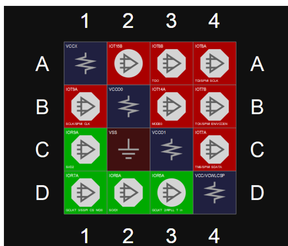
图 3-1 GW1NZ-1 器件 CS16 封装管脚分布示意图（顶视图）
