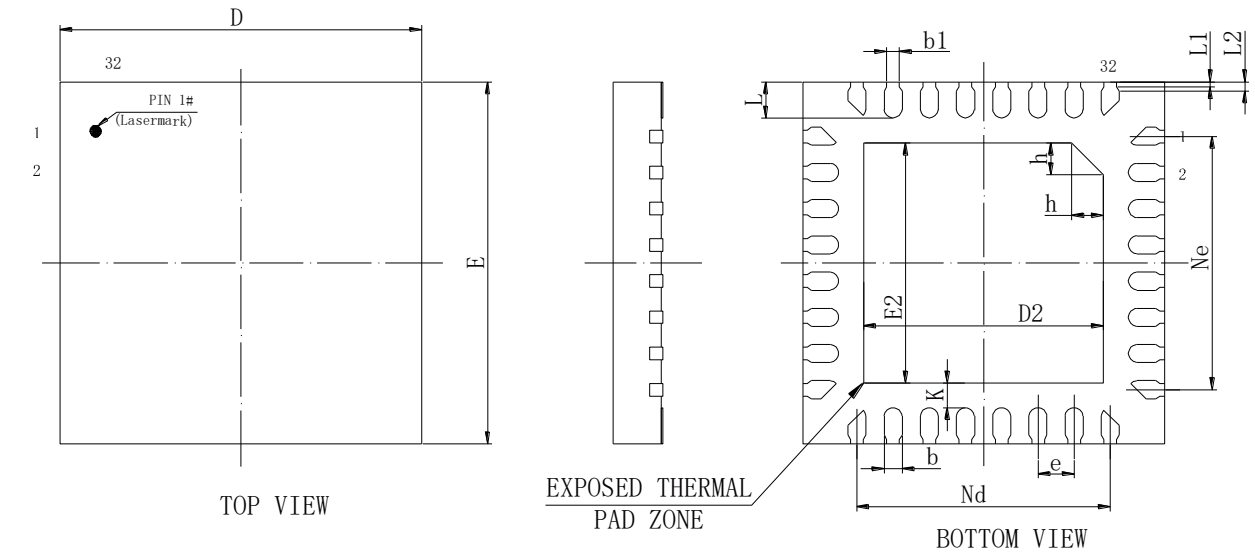
图 4-4 封装尺寸 FN32F
