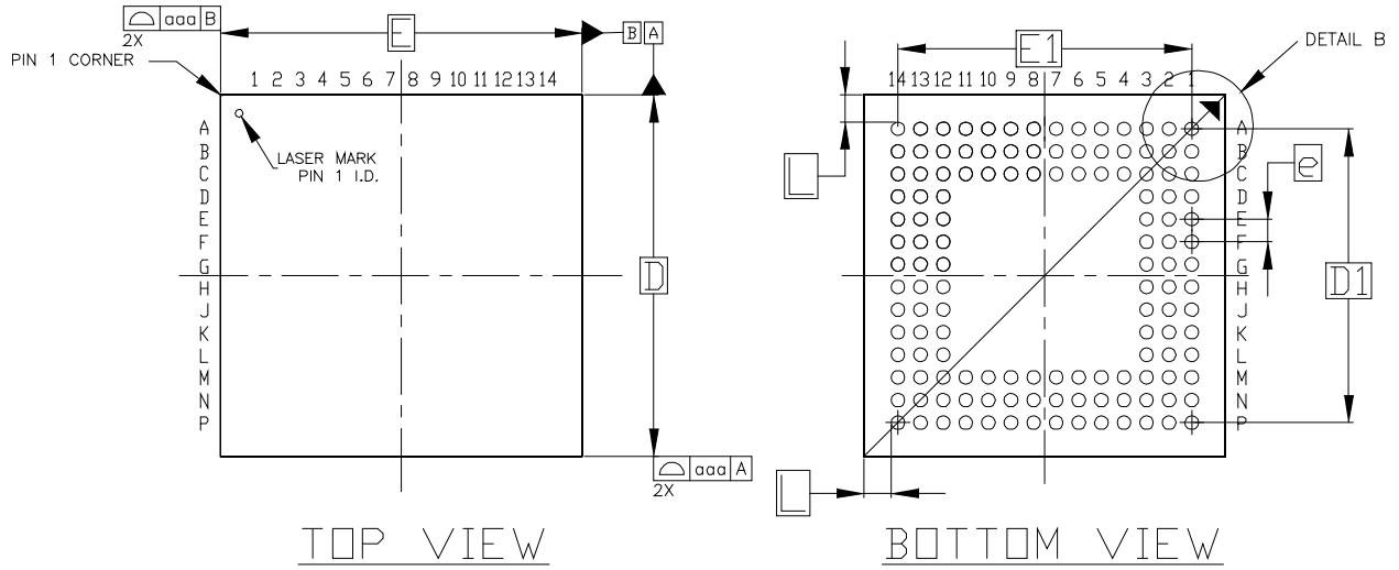
图 4-8 封装尺寸 MG132X
