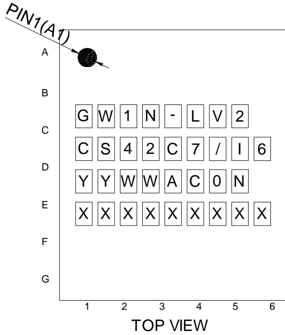
图 4-2 封装尺寸 CS42
