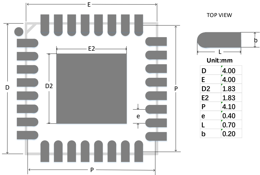
图 4-4 推荐 PCB Layout FN32
