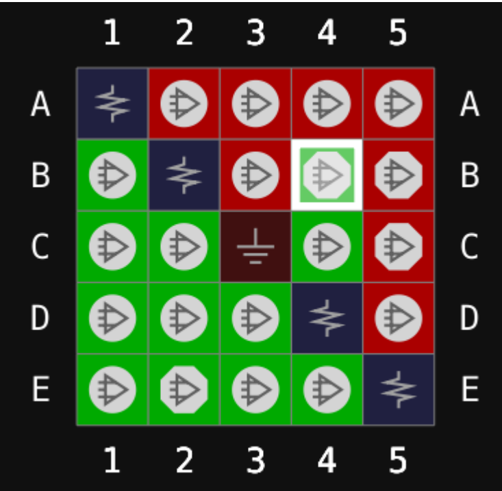
图 3-5 GW1NZ-1 器件 CG25 封装管脚分布示意图（顶视图）
