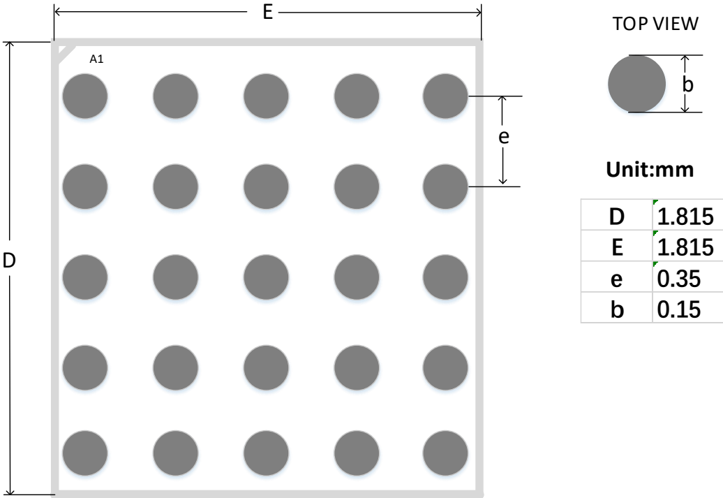
图 4-12 推荐 PCB Layout CG25
