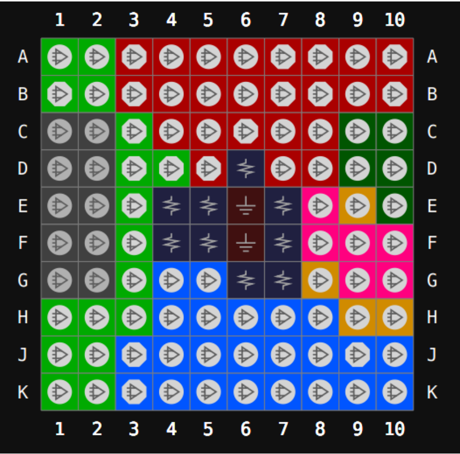
图 3-8 GW1NZ-2 器件 CS100H 封装管脚分布示意图（顶视图）
