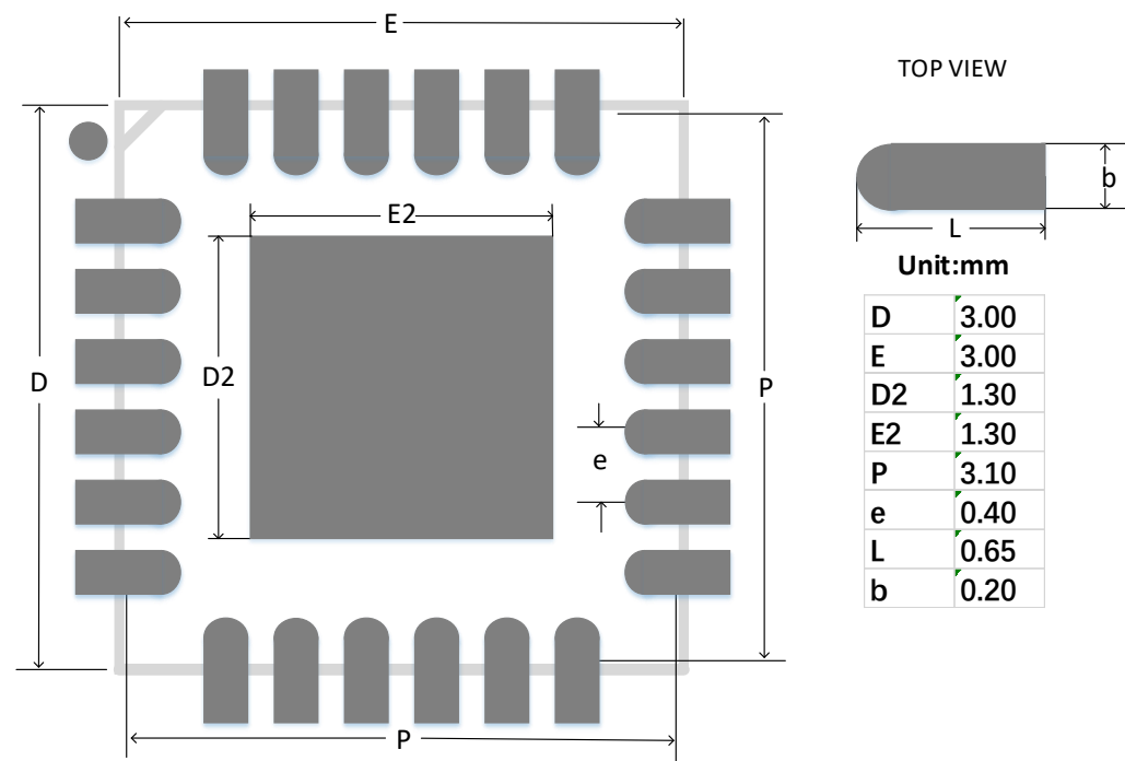
图 4-14 推荐 PCB Layout FN24
