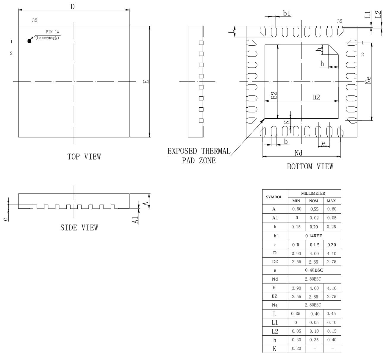
图 4-5 封装尺寸 FN32F
