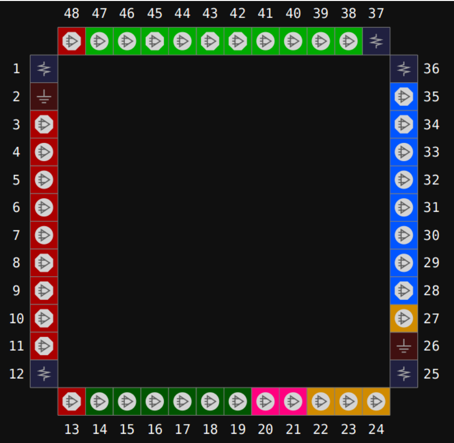
图 3-7 GW1NZ-2 器件 QN48 封装管脚分布示意图（顶视图）
