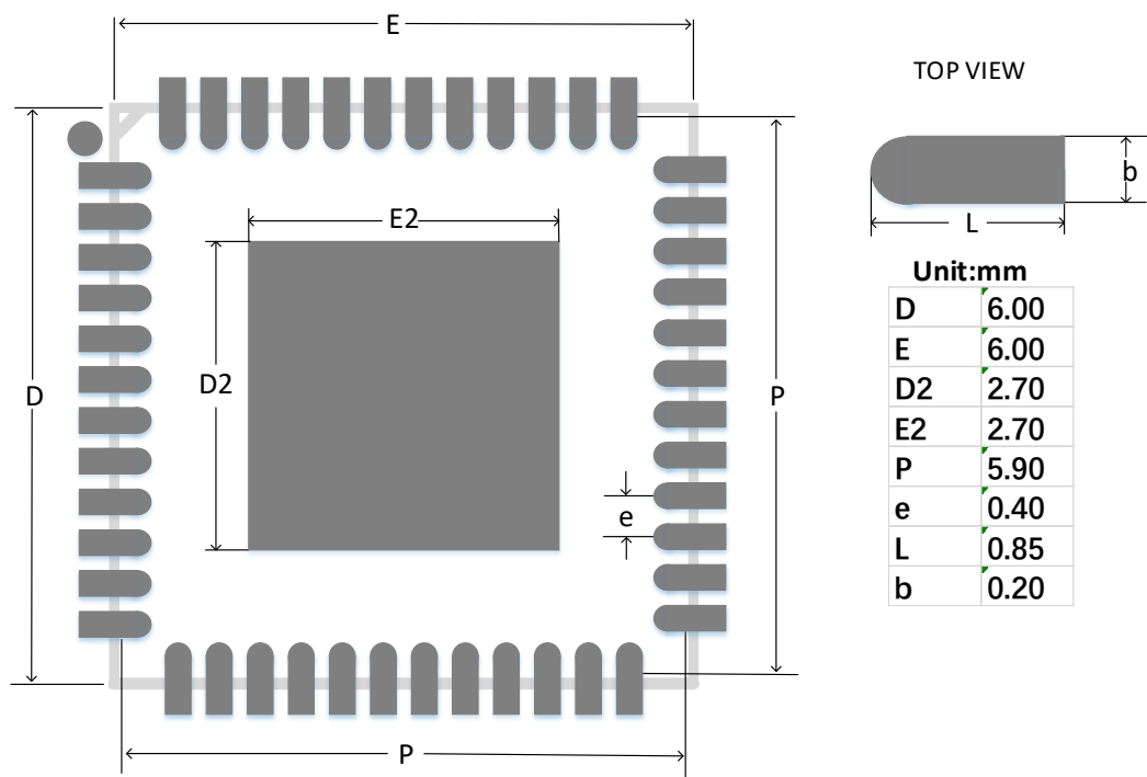
图 4-8 推荐 PCB Layout QN48
