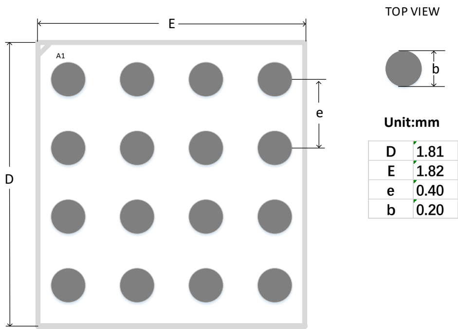
图 4-2 推荐 PCB Layout CS16
