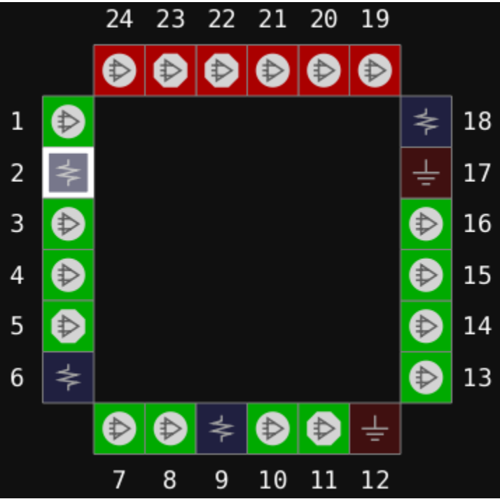
图 3-6 GW1NZ-1 器件 FN24 封装管脚分布示意图（顶视图）
