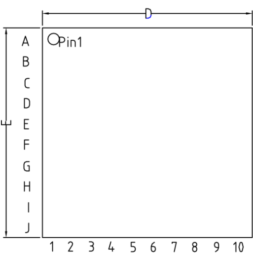
图 4-9 封装尺寸 CS100H
