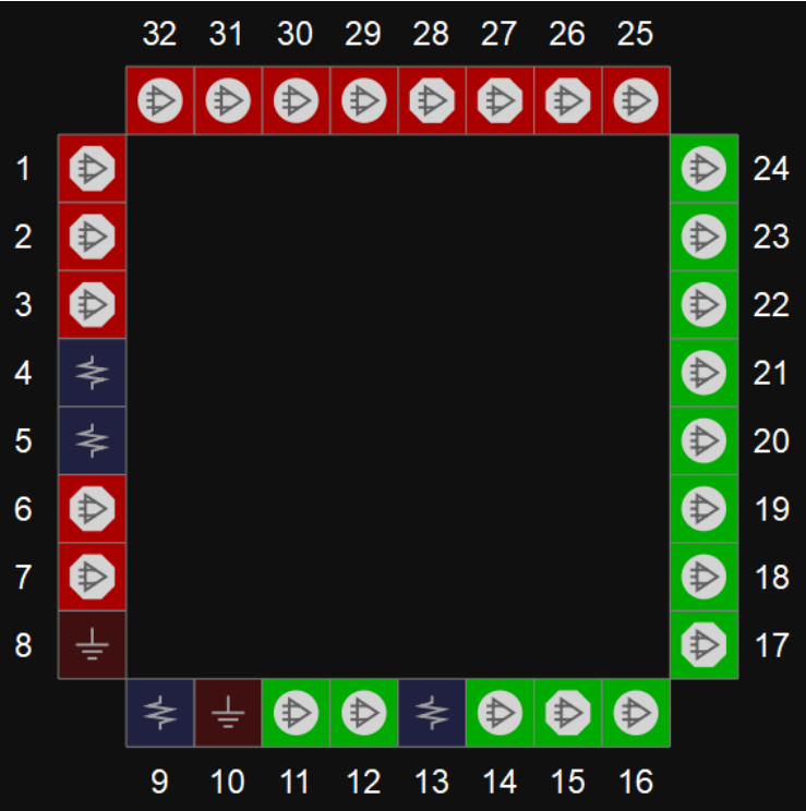
图 3-2 GW1NZ-1 器件 FN32 封装管脚分布示意图（顶视图）
