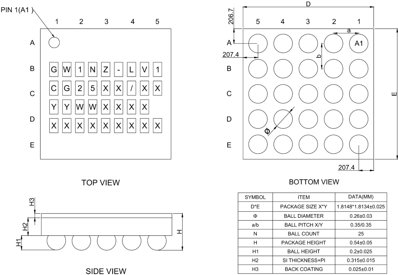
图 4-11 封装尺寸 CG25
