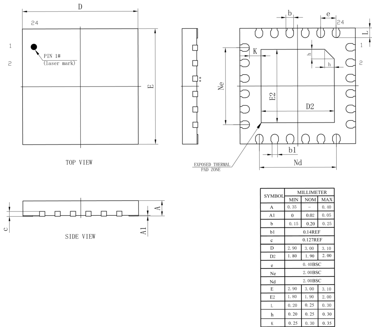
图 4-13 封装尺寸 FN24
