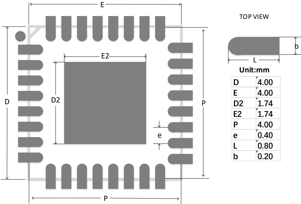
图 4-6 推荐 PCB Layout FN32F
