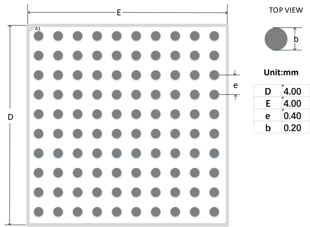
图 4-10 推荐 PCB Layout CS100H
