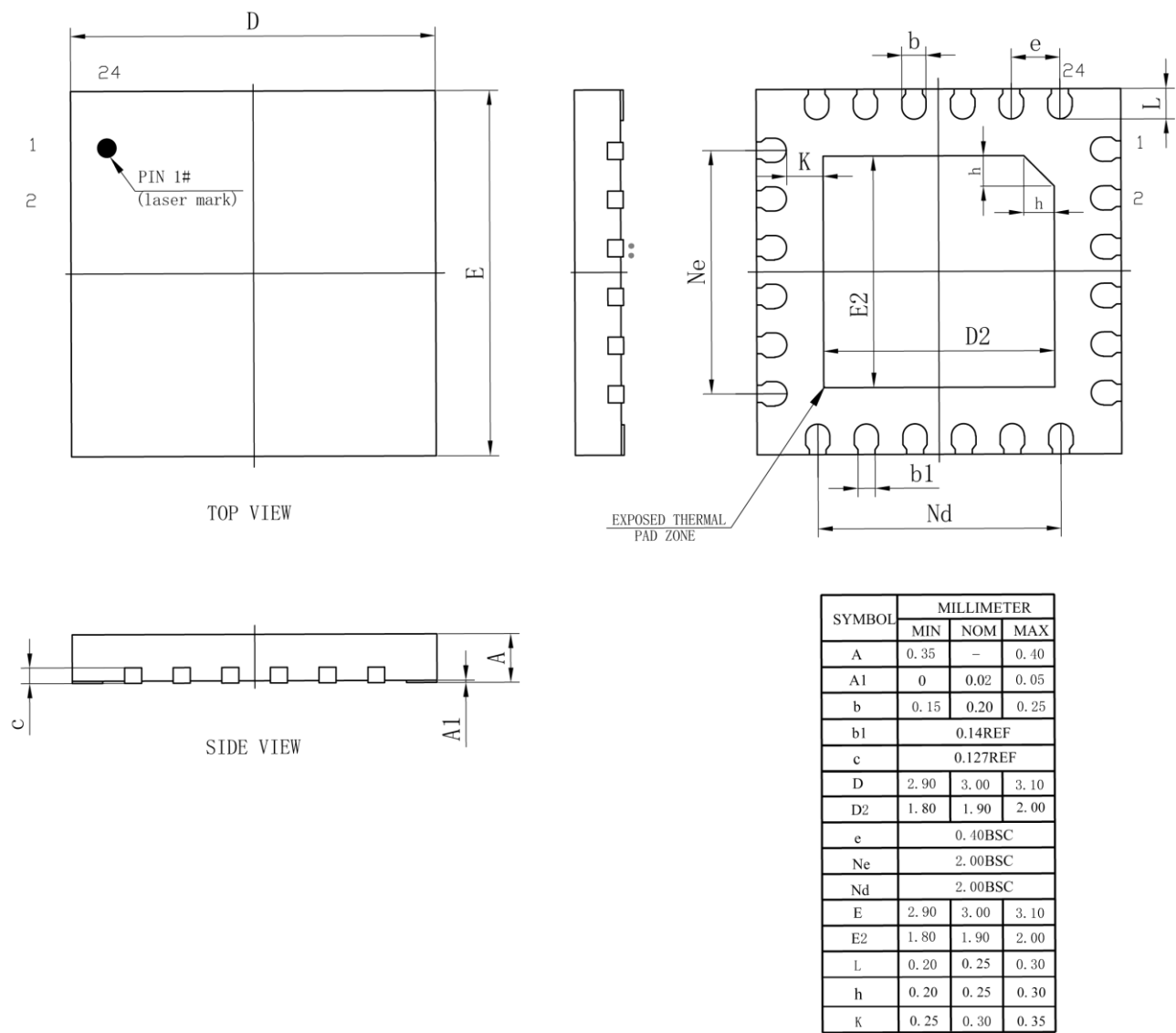
图 4-13 封装尺寸 FN24
