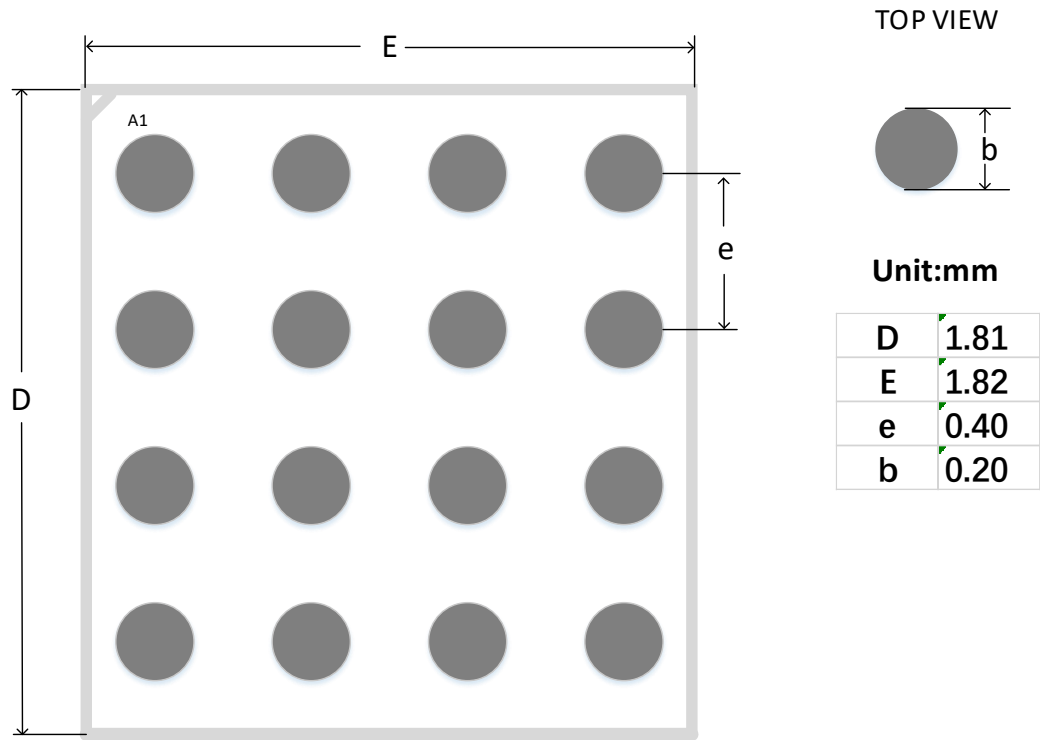
图 4-2 推荐 PCB Layout CS16
