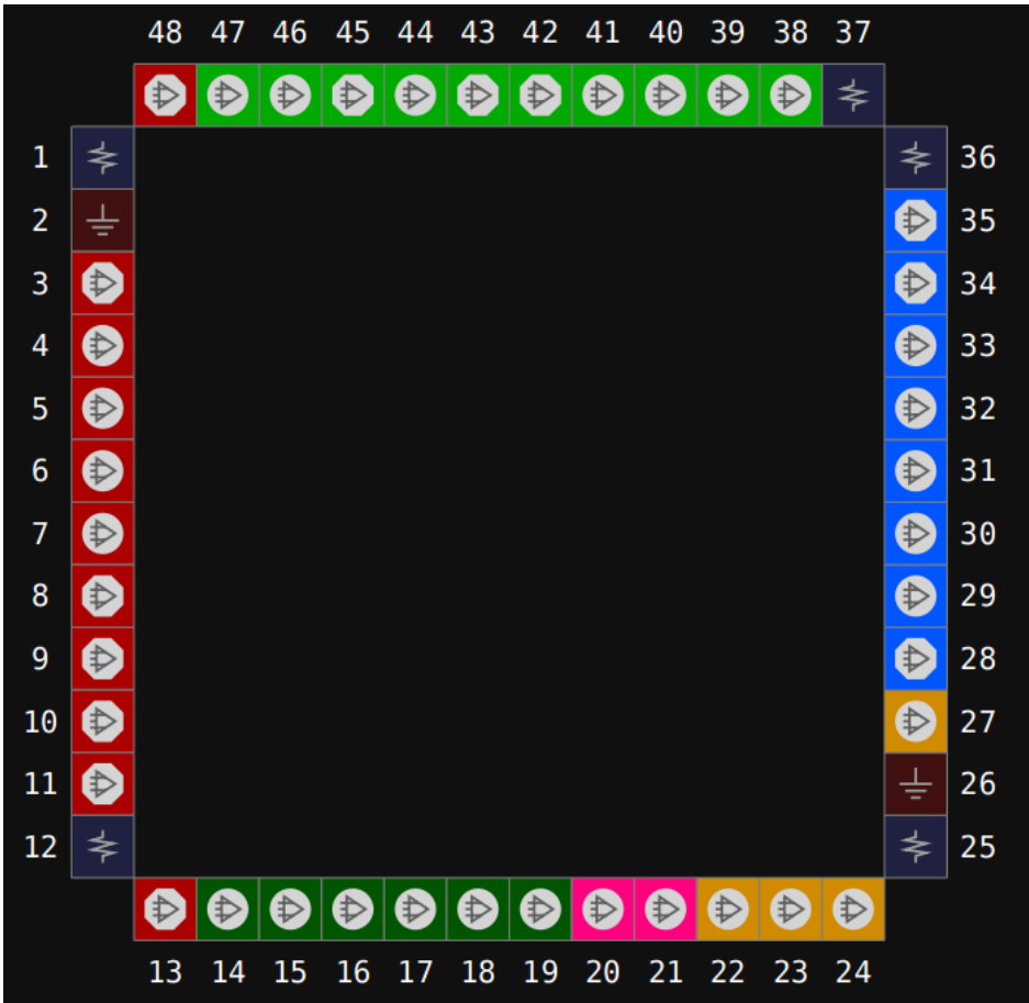
图 3-7 GW1NZ-2 器件 QN48 封装管脚分布示意图（顶视图）
