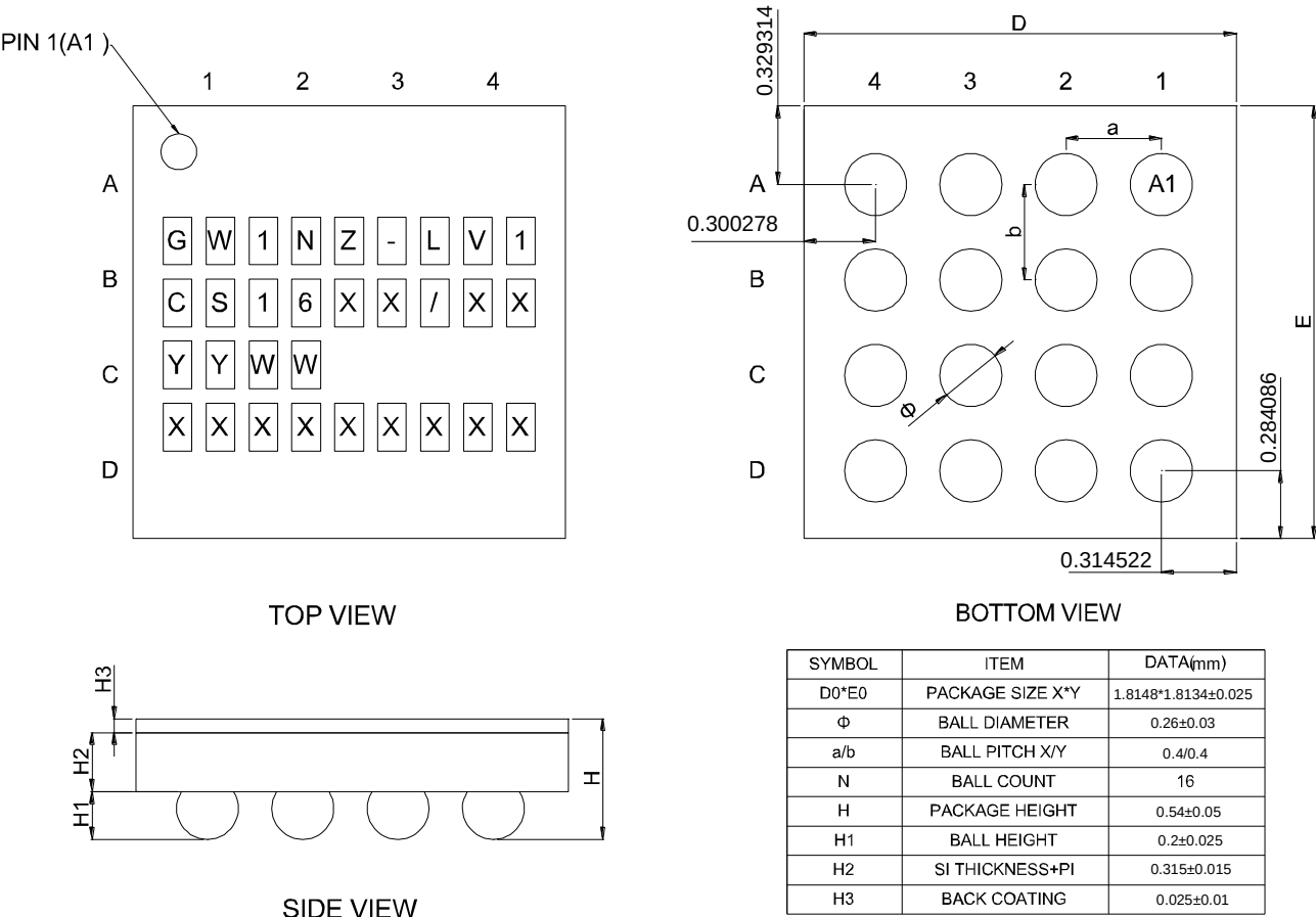
图 4-1 封装尺寸 CS16
