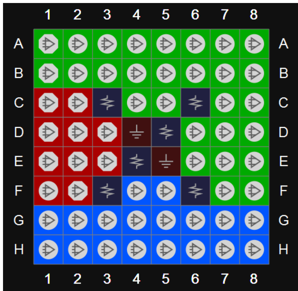
图 3-4 GW1NSR-4/GW1NSR-4C 器件 MG64P 封装管脚分布示意图（顶视图）
