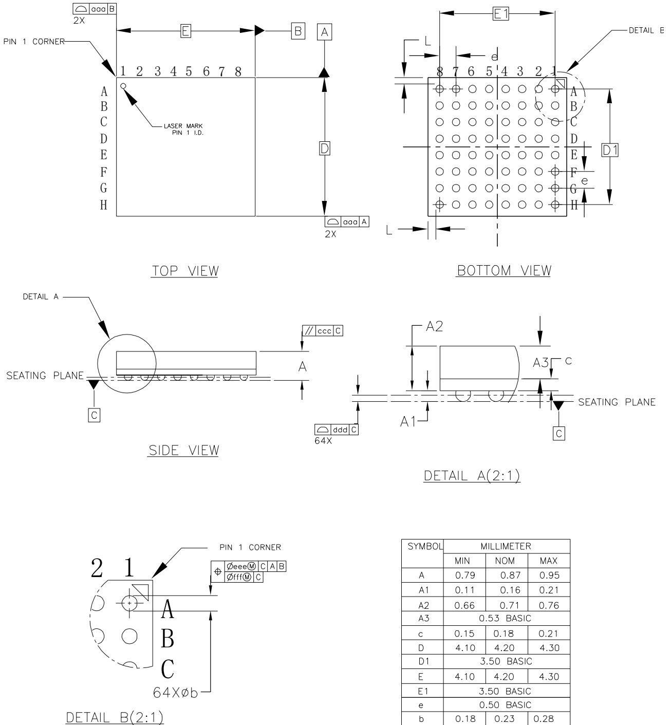
图 4-3 封装尺寸 MG64P
