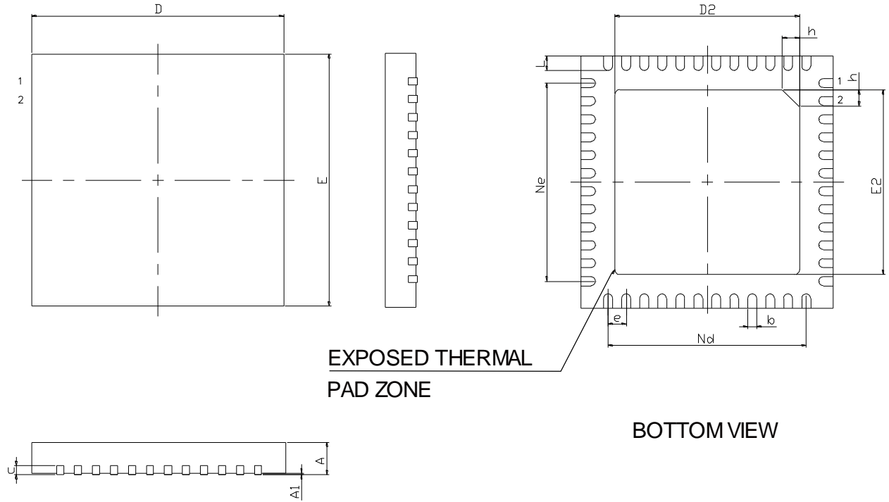
图 4-1 封装尺寸 QN48
