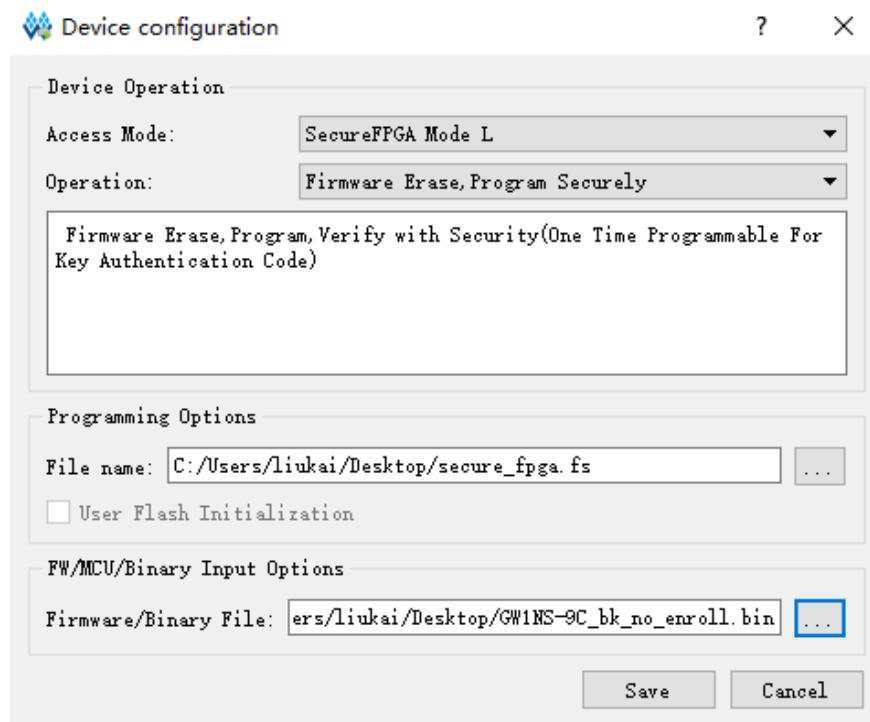
图 2-8 GW1NE-9C (Gowin_EMPU_M1)下载属性配置
