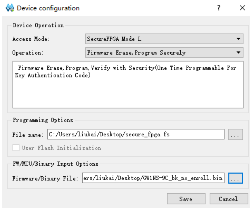
图 3-11 GW1NE-9C (Gowin_EMPU_M1)下载属性配置
