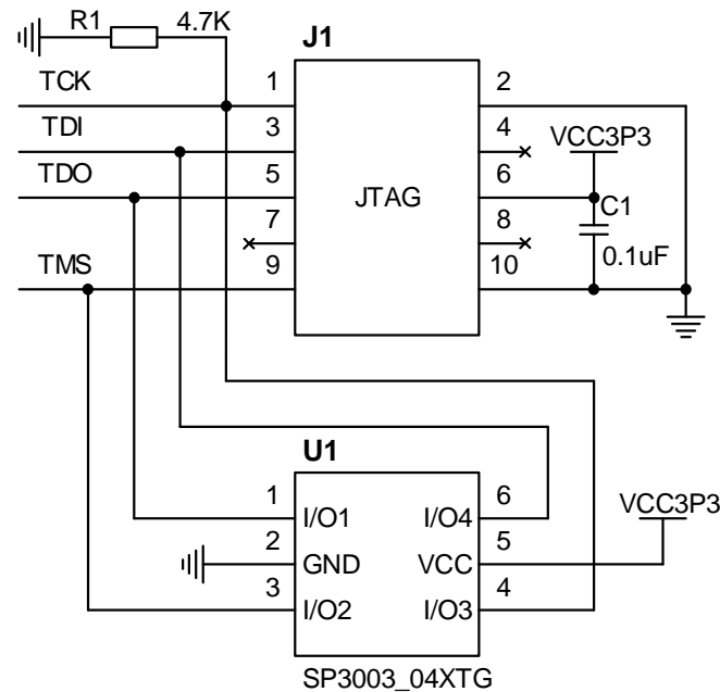
图 3 JTAG 电路
