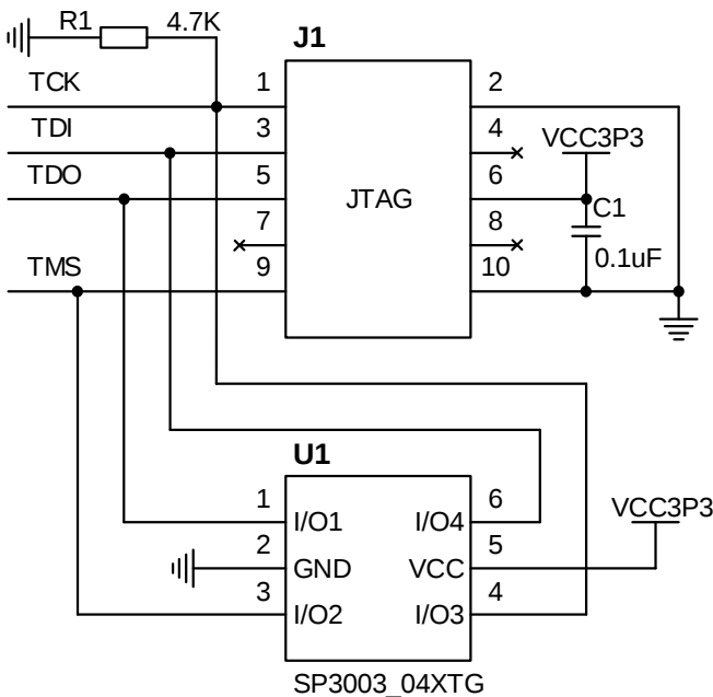
图 3 JTAG 电路
