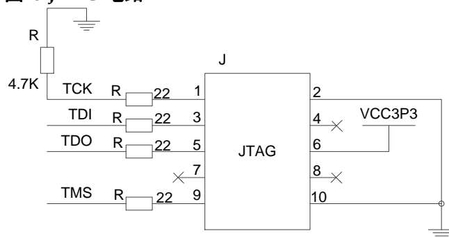
图 3 JTAG 电路
