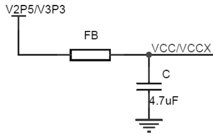
图 2 LV 版 VCC 核电压输入端噪声处理
