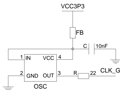
图 8 FPGA 外接晶振电路
