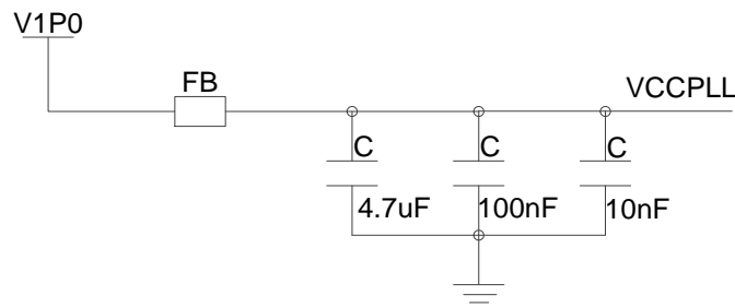
图 4 隔离滤波 V CC PLL
