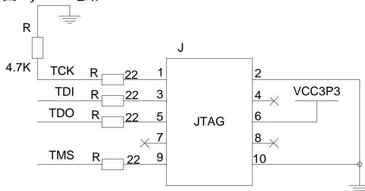
图 5 JTAG 电路
