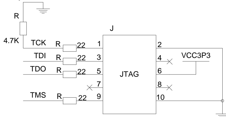
图 5 JTAG 电路
