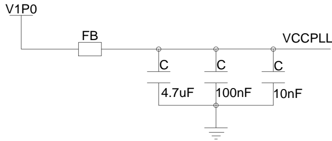
图 4 隔离滤波 V CCPLL
