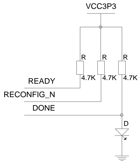
图 6 READY、RECONFIG_N、DONE 参考电路
