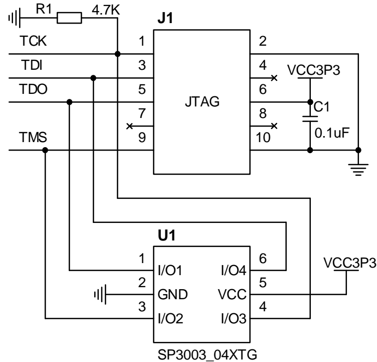
图 5 JTAG 电路
