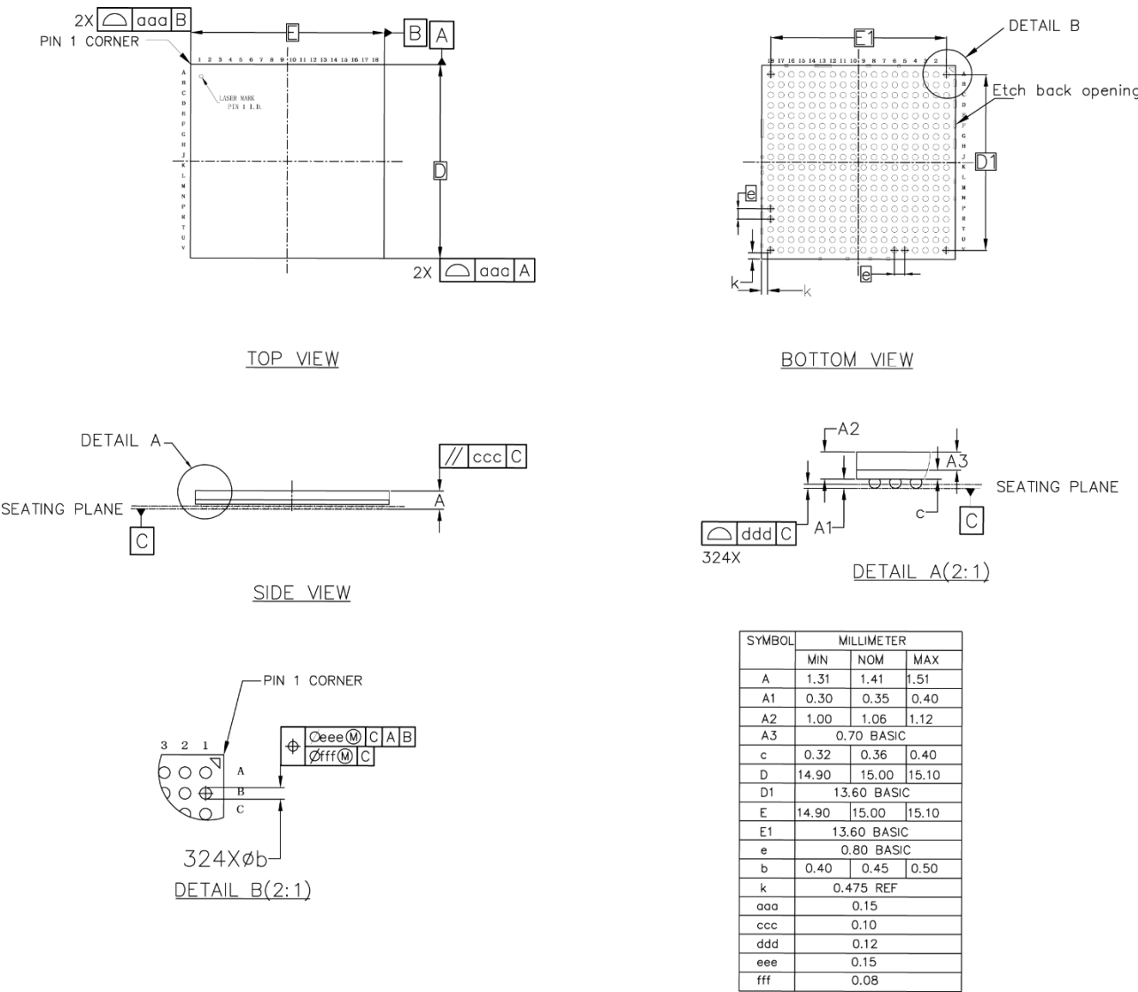
图 4-11 封装尺寸 UG324A
