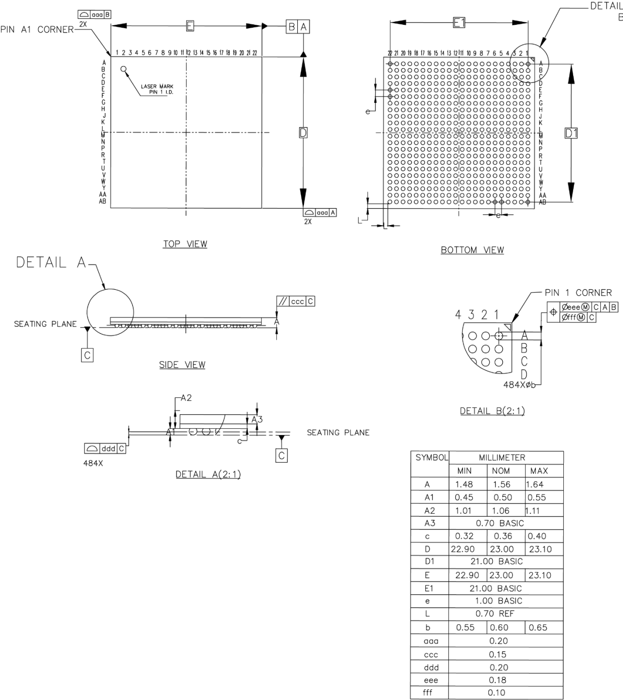
图 4-5 封装尺寸 PG484
