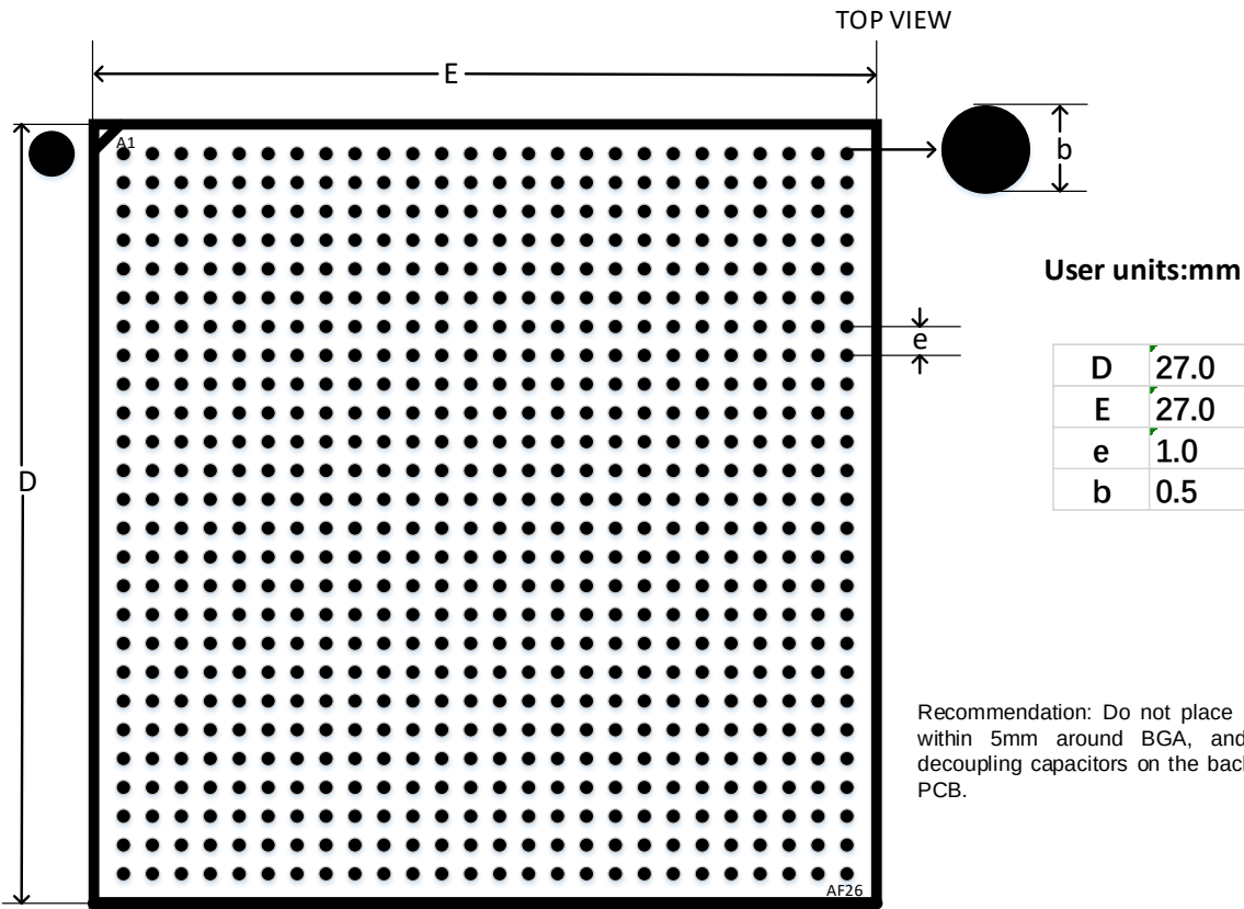
图 4-2 推荐 PCB Layout
