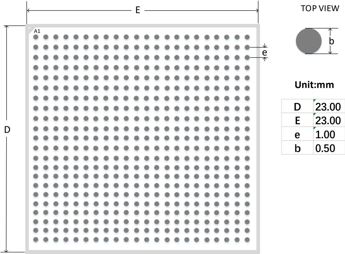
图 4-6 推荐 PCB Layout
