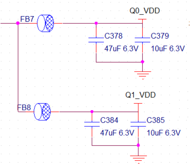
图 2-2 磁珠隔离
