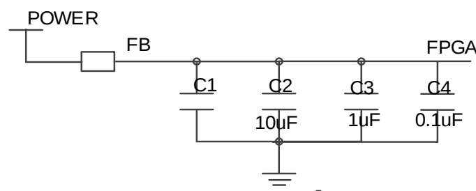
图 2-1 隔离滤波
