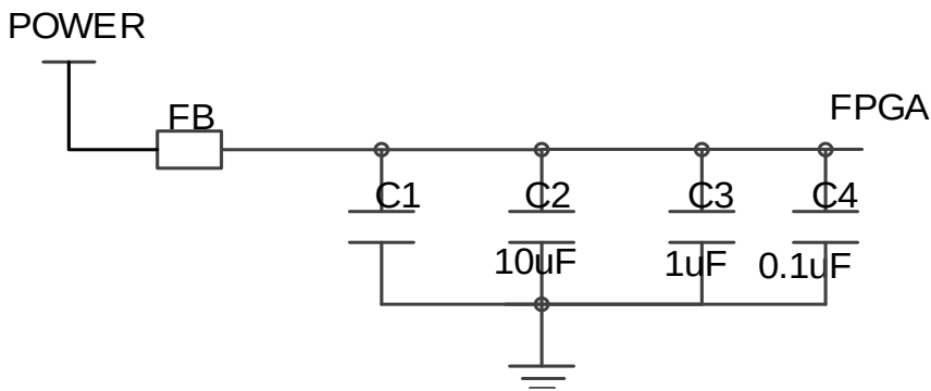
图 2-1 隔离滤波
