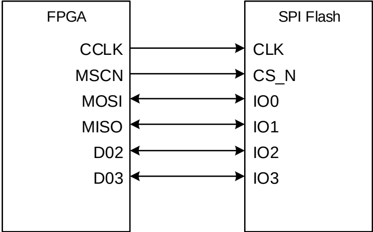
图 4-4 MSPIx4 配置模式连接示意图
