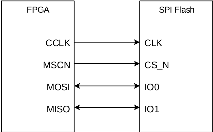
图 4-3 MSPIx2 配置模式连接示意图
