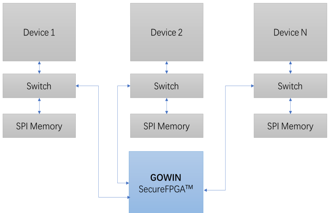
图 5 Gowin SecureFPGA™ 服务器应用的安全启动
