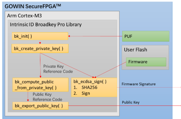
图 3 SecureFPGA™ - 安全启动准备
