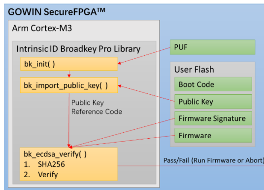
图 4 SecureFPGA™ - 安全启动验证
