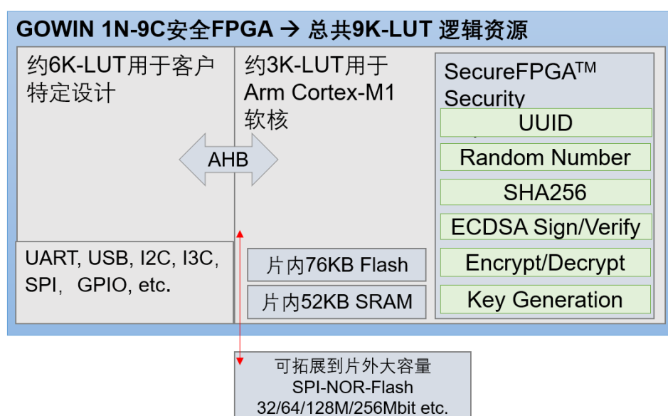
图 1 GWIN-9C SecureFPGA™ 器件
