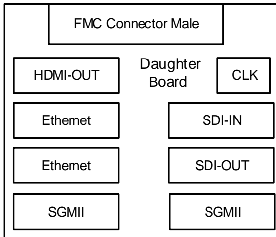
图 3-4 系统框图
