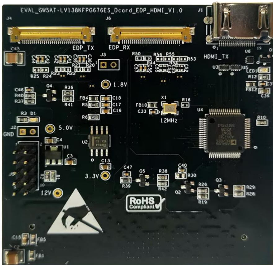
图 6-1 EVAL_GW5AT-LV138KFG676ES_Dcard_EDP_HDMI_V1.0 子板
