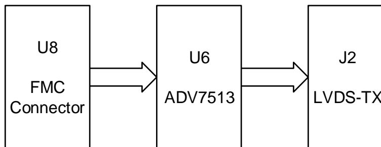
图 3-7 HDMI-TX 接口连接示意图
