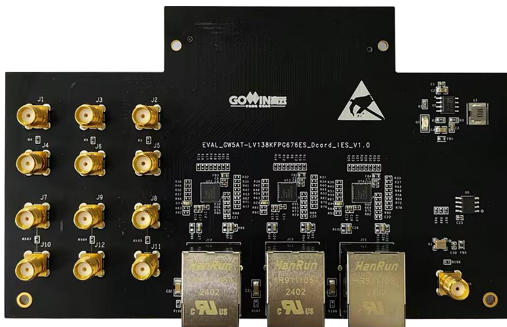
图 2-1 EVAL_GW5AT-LV138KFPG676ES_Dcard_IES_V1.0 子板
