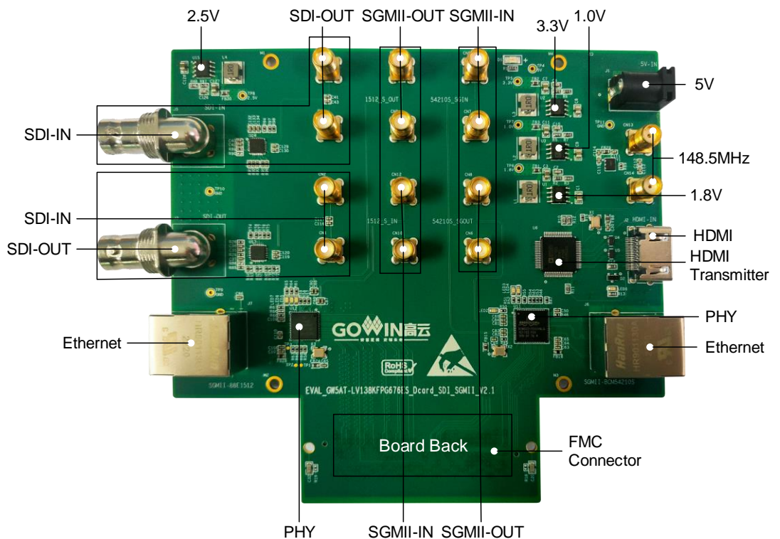
图 3-3 子板 PCB 组件说明
