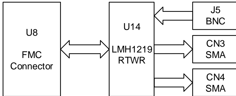
图 3-9 SDI-OUT 接口连接示意图
