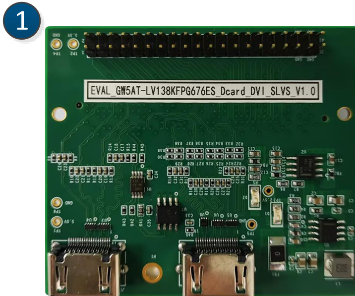
① EVAL_GW5AT-LV138KFPG676ES_Dcard_DVI_SLVS_V1.0子板
