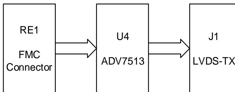
图 6-8 HDMI-TX 接口连接示意图
