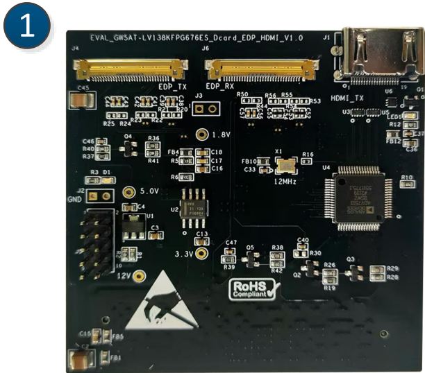
① EVAL_GW5AT-LV138KFG676ES_Dcard_EDP_HDMI_V1.0子板
