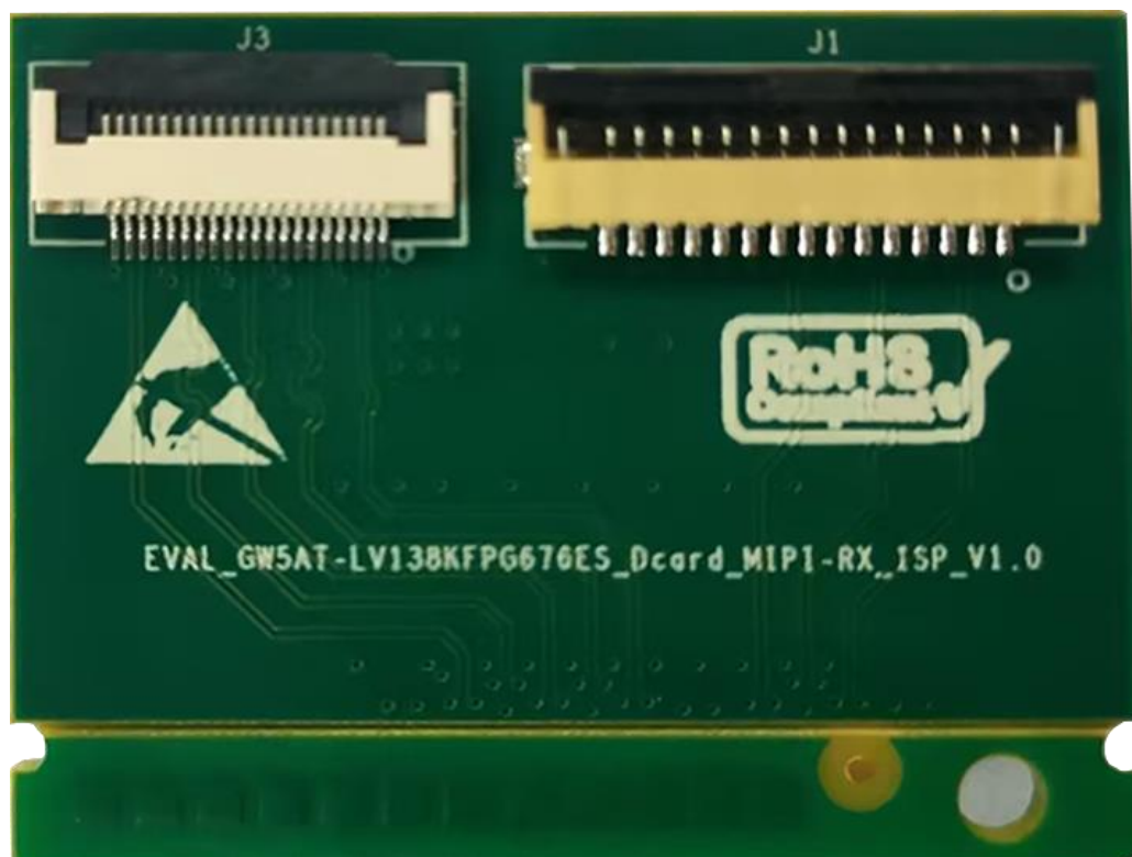
图 4-1 EVAL_GW5AT-LV138KFPG676ES_Dcard_MIPI-RX_ISP_V1.0 子板
