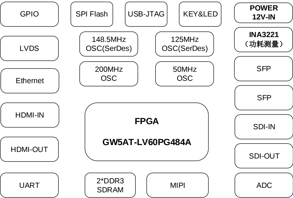
图 2-4 系统框图
