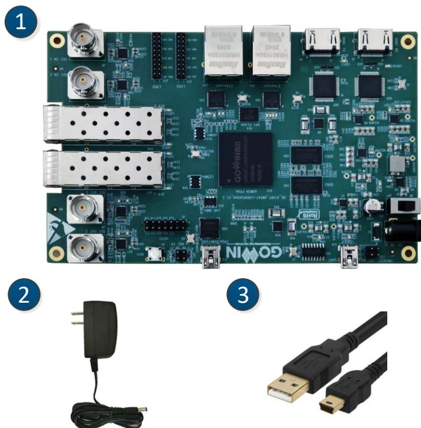
图 2-2 开发板套件
