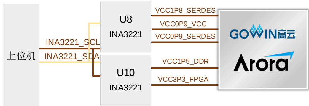
图 3-14 I2C 接口连接示意图
