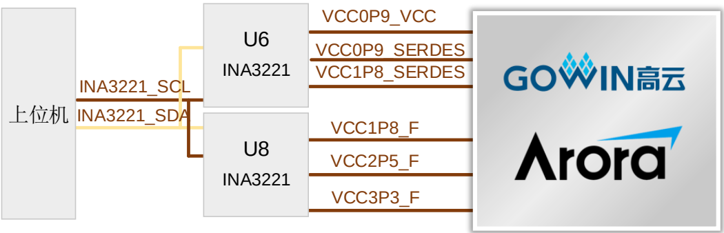
图 3-4 I2C 接口连接示意图
