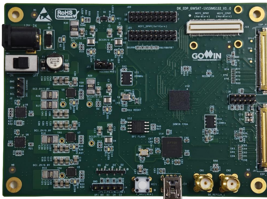
图 2-1 DK_EDP_GW5AT-LV15MG132_V1.0 开发板
