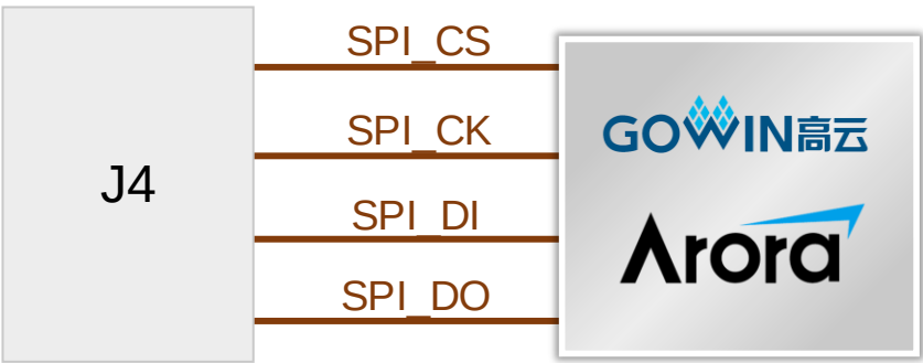
图 3-7 SPI 接口连接示意图
