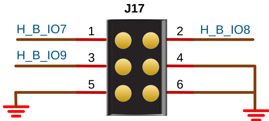
图 3-7 GPIO 电路
