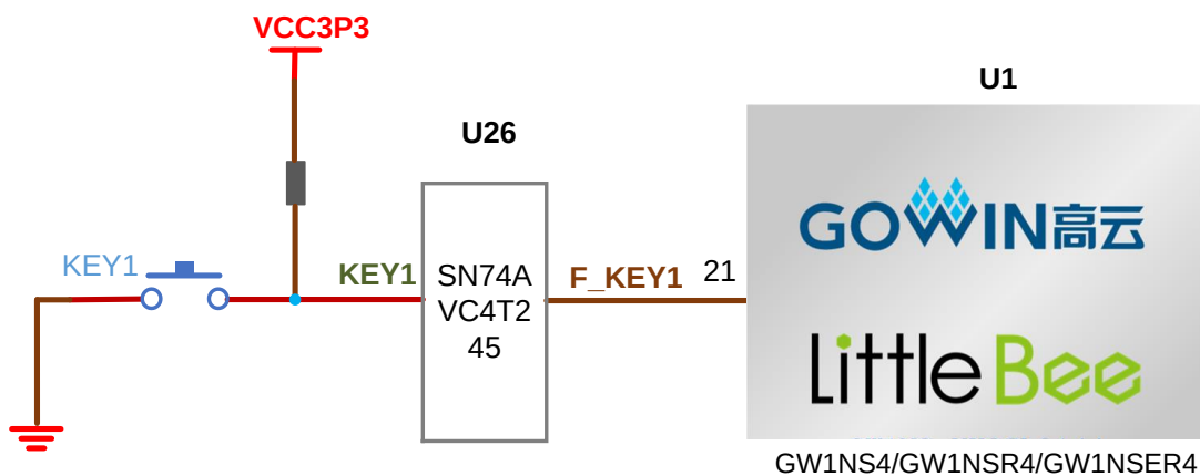
图 3-6 按键电路
