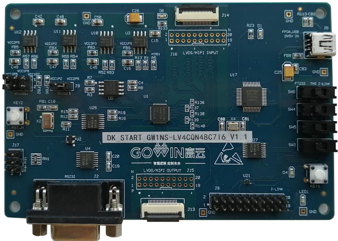
图 2-1 DK_START_GW1NS-LV4CQN48C7I6_V1.1 开发板
