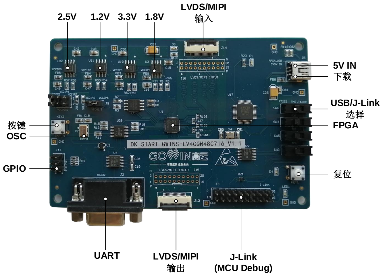
图 2-3 开发板 PCB 组件说明
