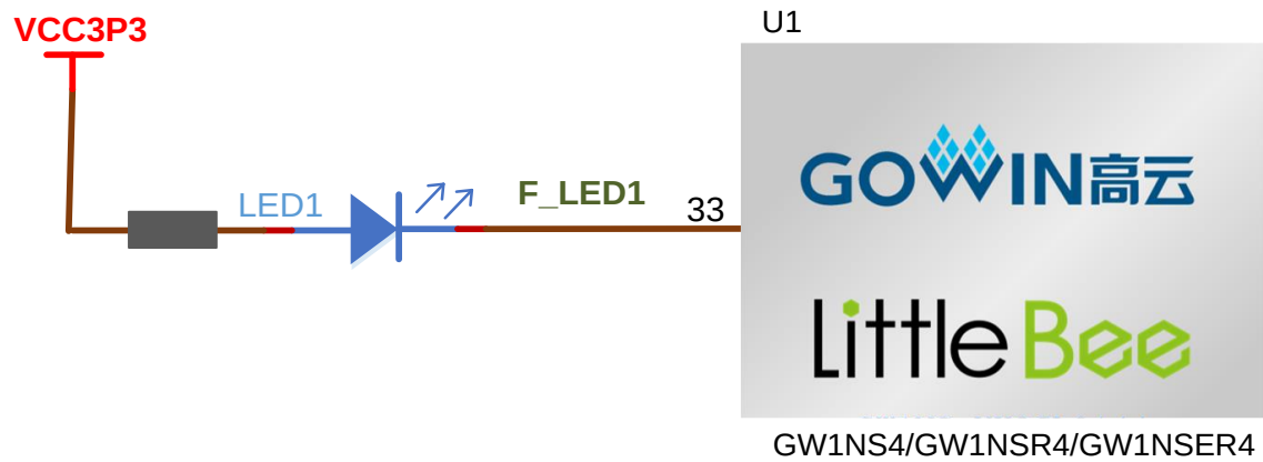
图 3-5 LED 电路
