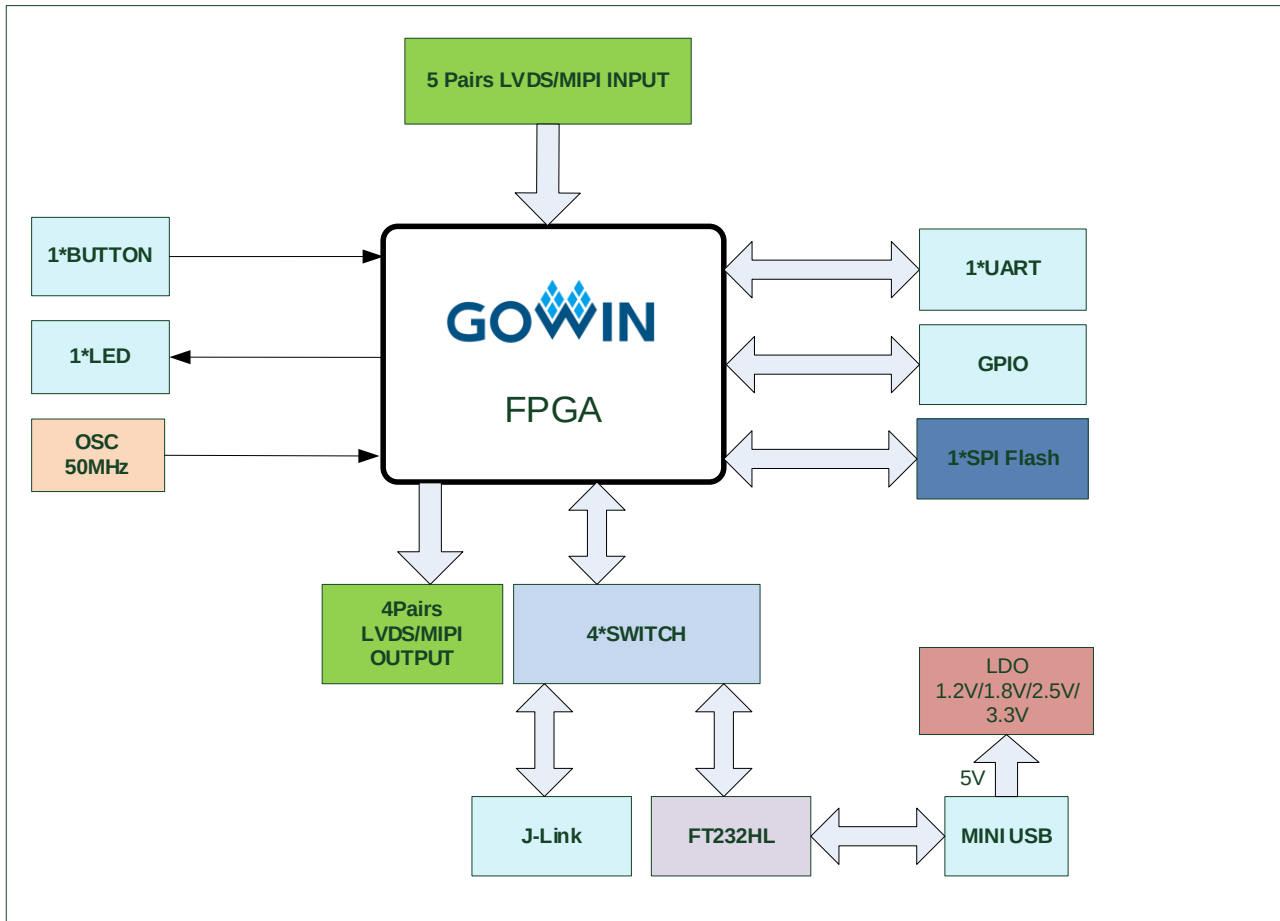
图 2-4 系统框图
