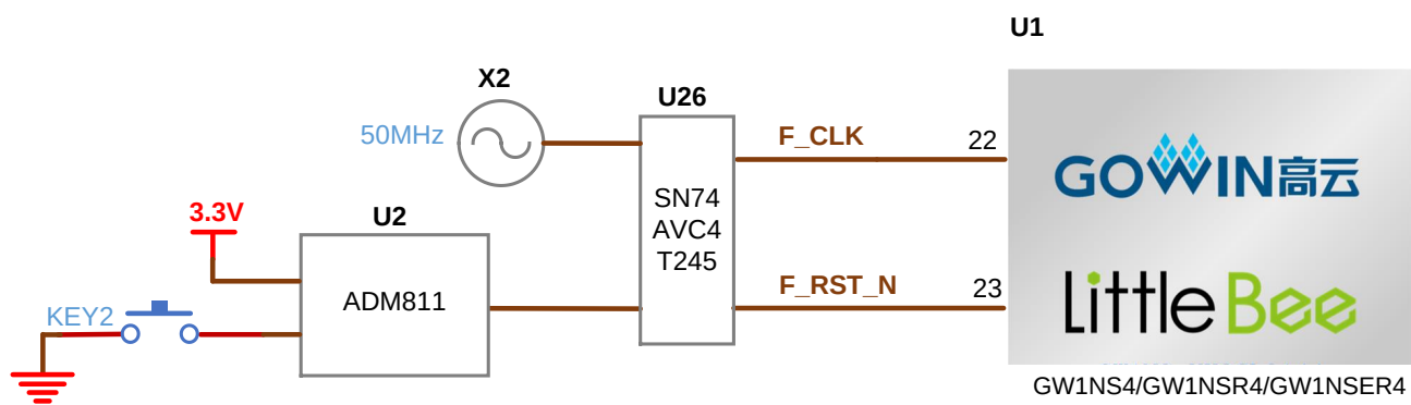
图 3-4 时钟、复位电路
