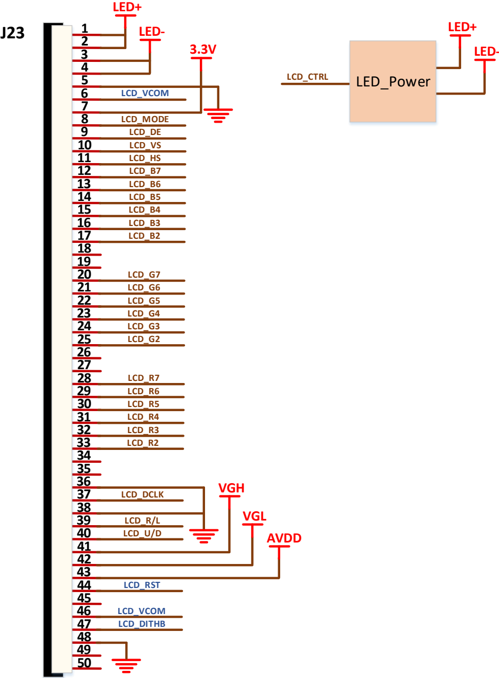
图 3-17 50pin FPC 接口示意图
