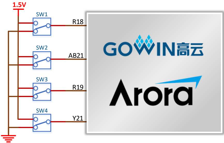
图 3-20 开关电路
