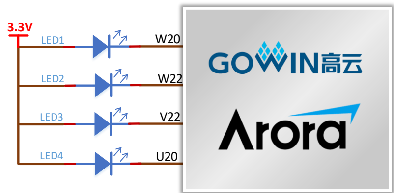
图 3-18 LED 连接示意图
