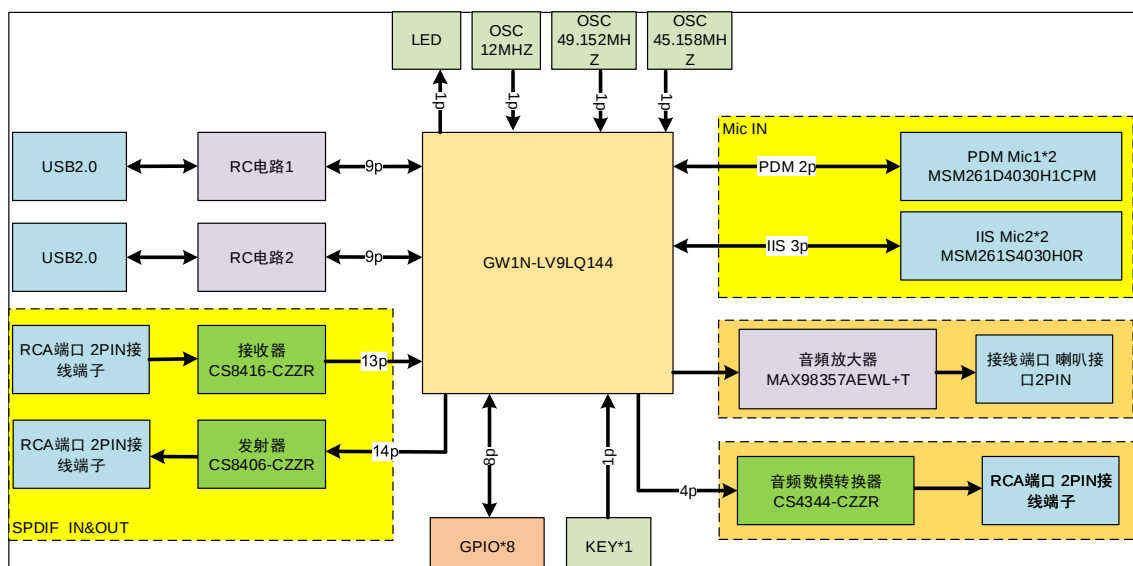
图 2-4 系统框图
