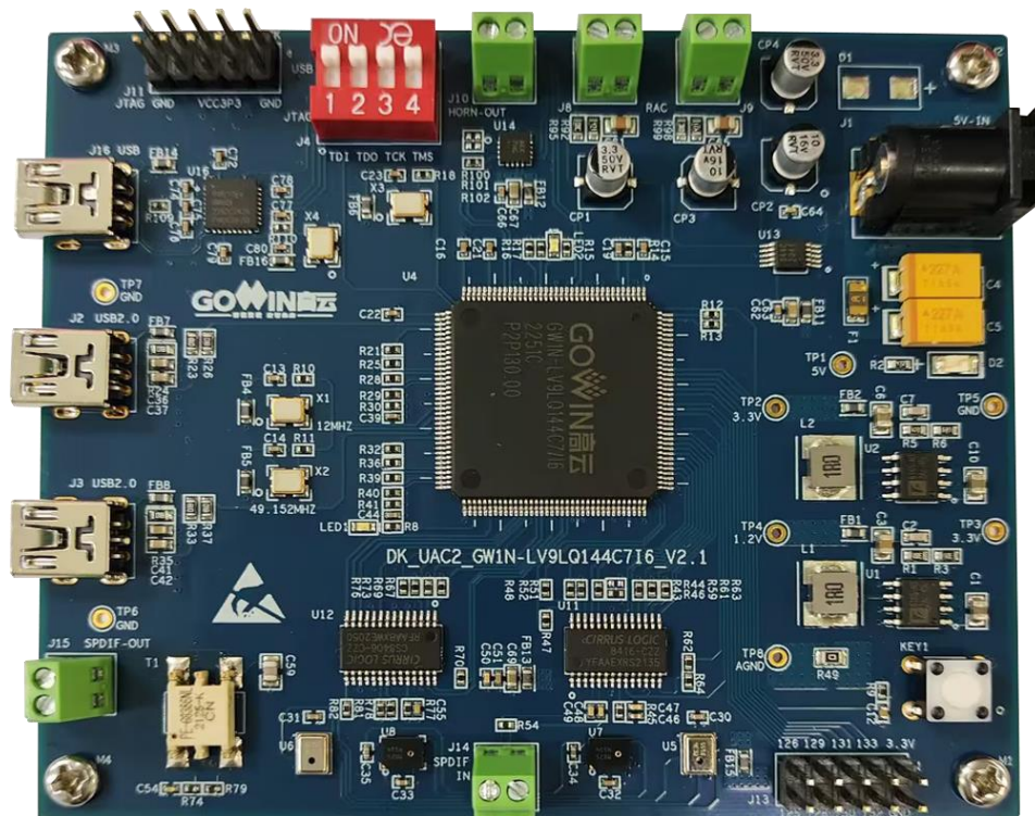
图 2-1 DK_UAC2_GW1N-LV9LQ144C7I6_V2.1 开发板
