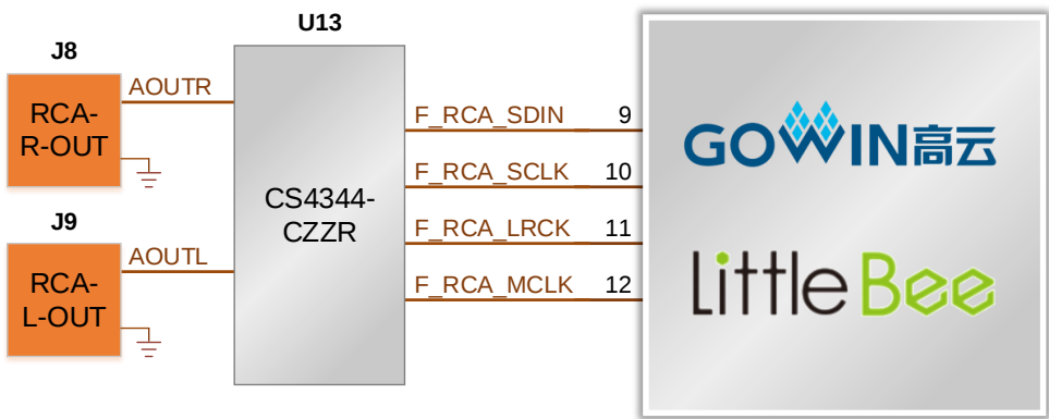
图 3-7 RCA 接口连接示意图
