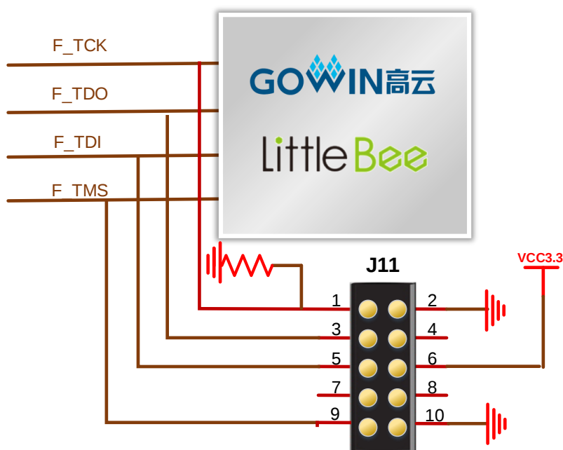
图 3-1 JTAG 下载连接示意图
