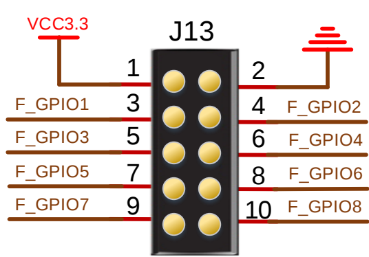
图 3-8 GPIO 连接示意图
