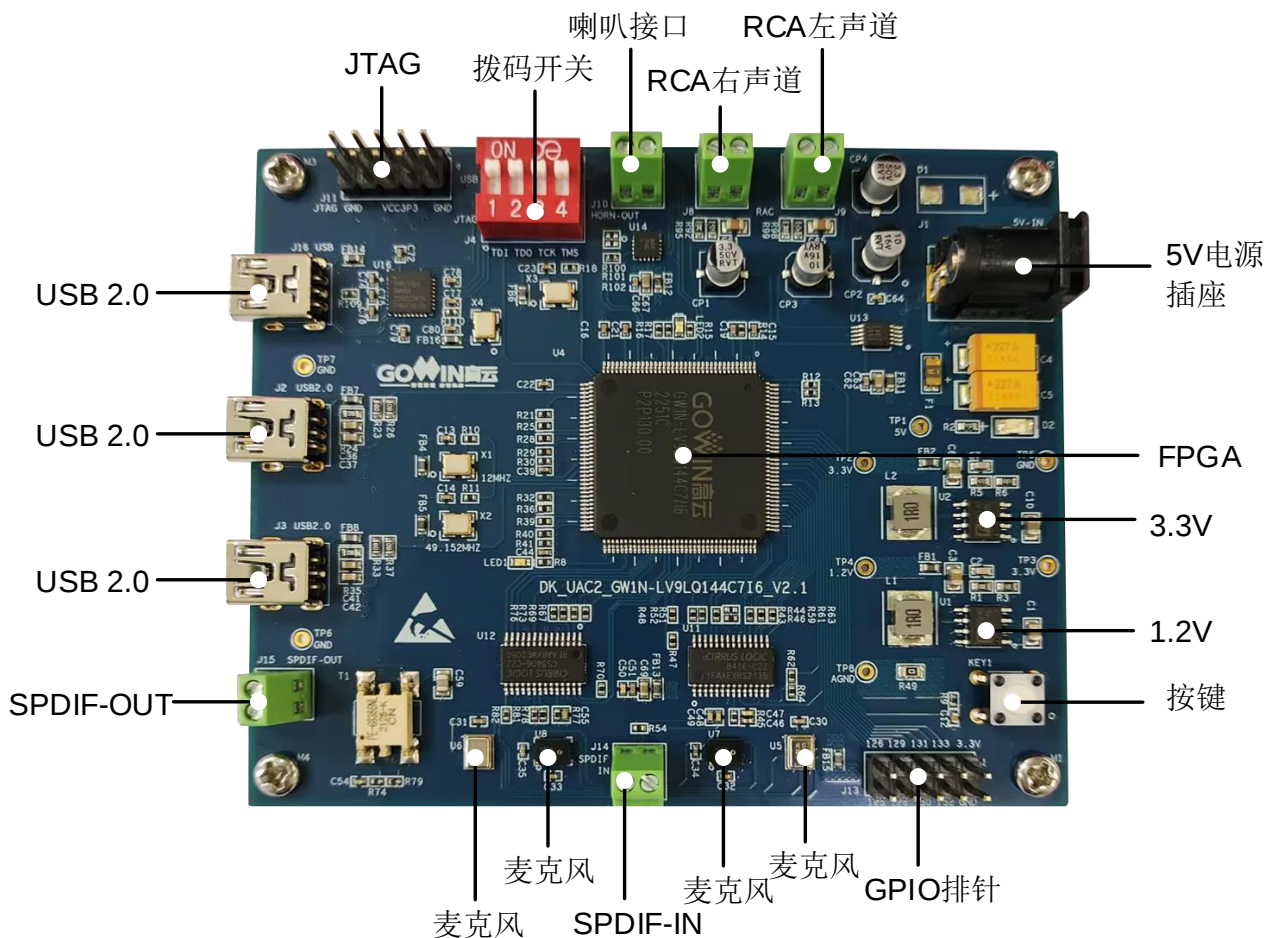
图 2-3 开发板 PCB 组件说明
