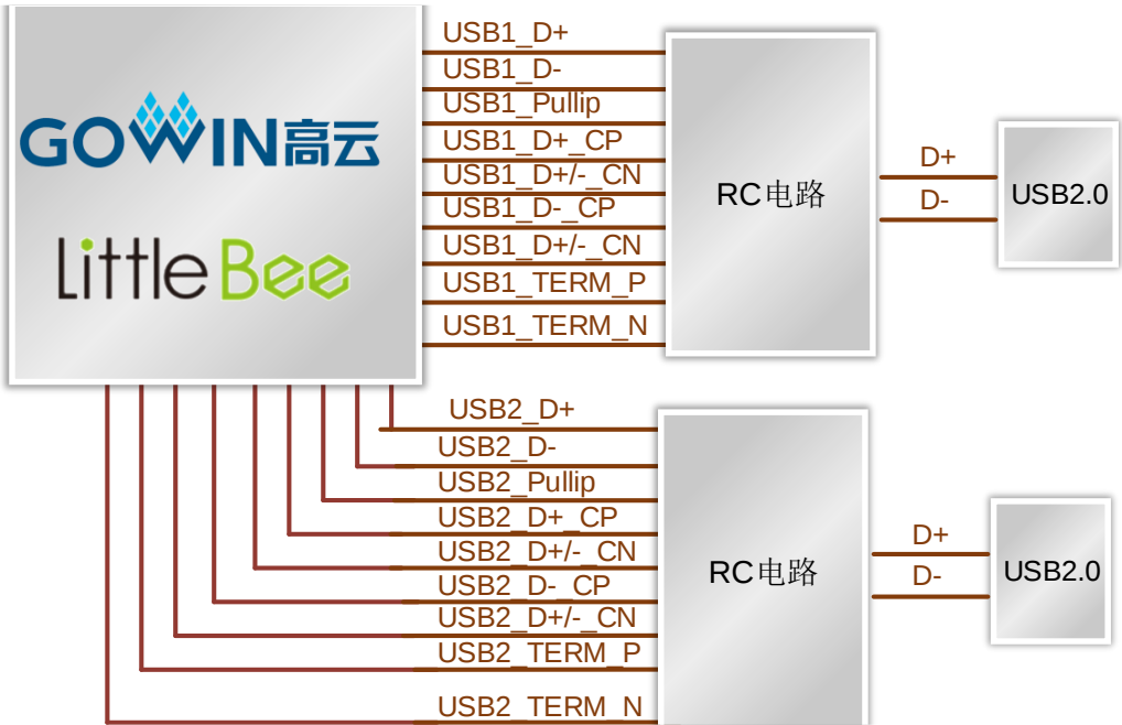
图 3-3 USB 接口连接示意图
