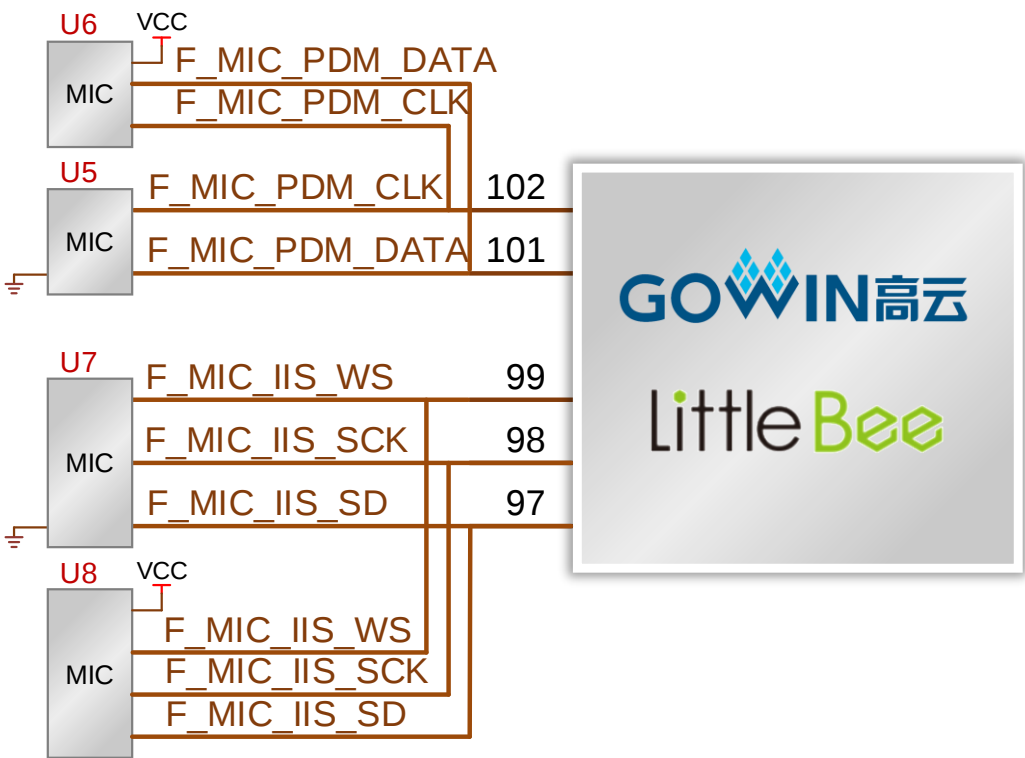
图 3-4 麦克风连接示意图
