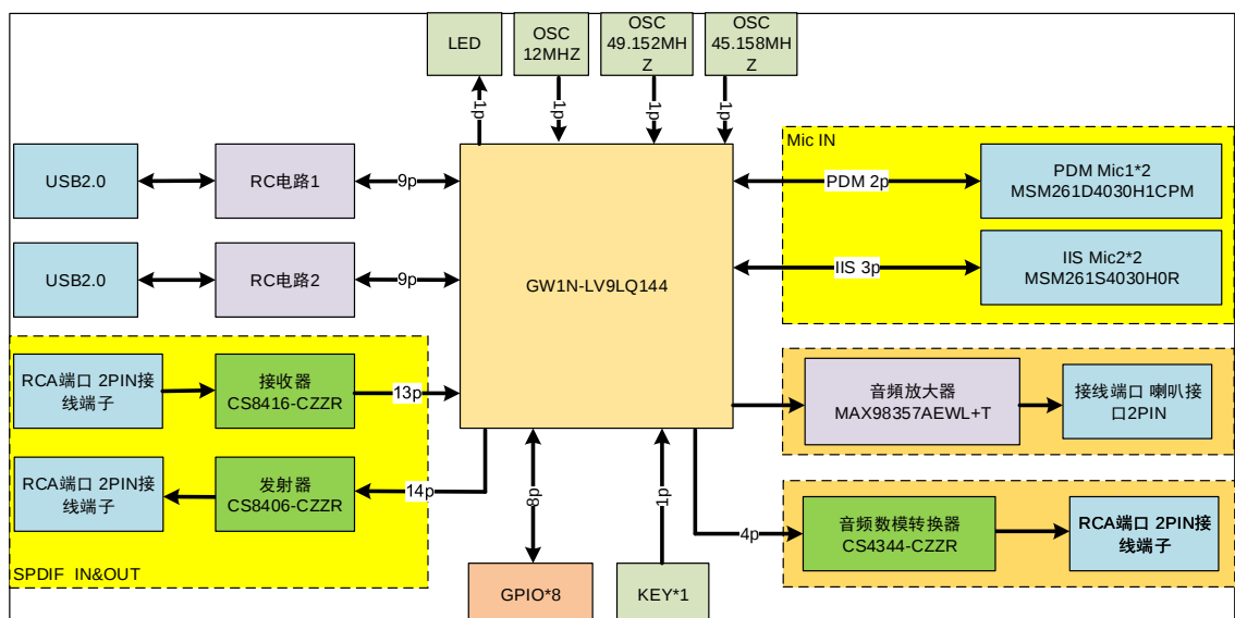
图 2-4 系统框图
