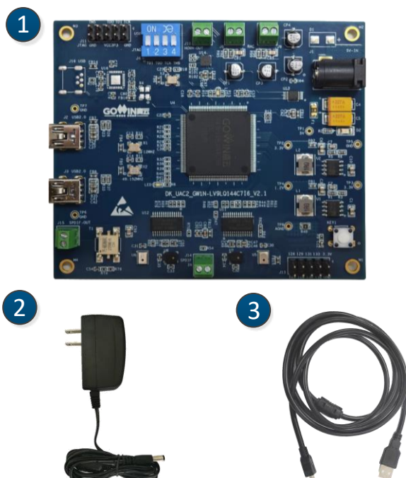
图 2-2 开发板套件
