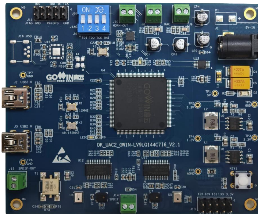
图 2-1 DK_UAC2_GW1N-LV9LQ144C7I6_V2.1 开发板
