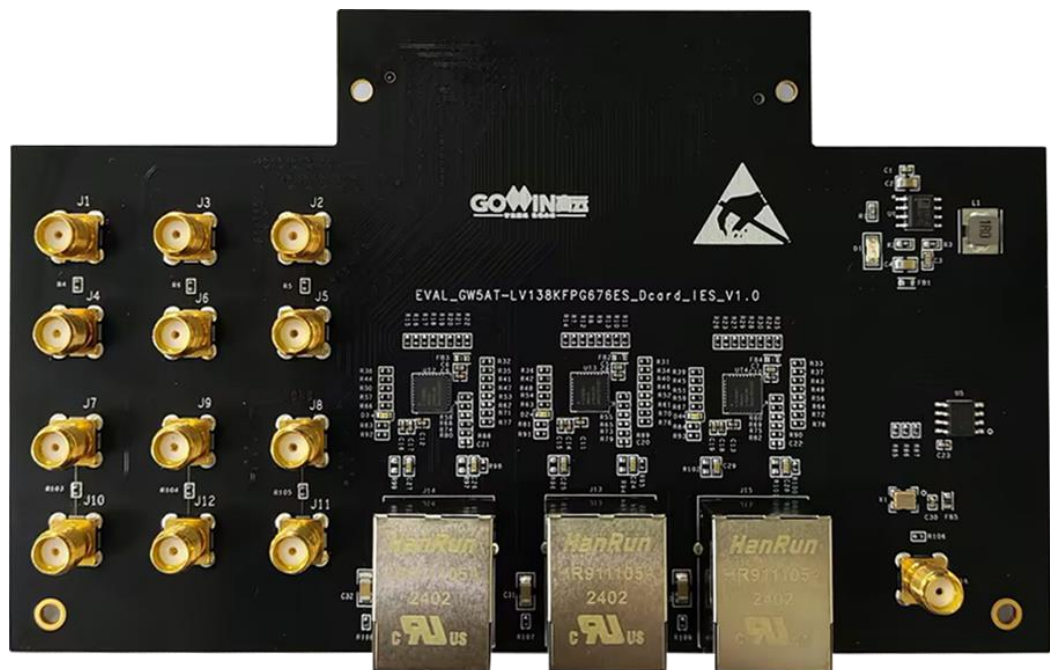
图 2-1 EVAL_GW5AT-LV138KFPG676ES_Dcard_IES_V1.0 子板
