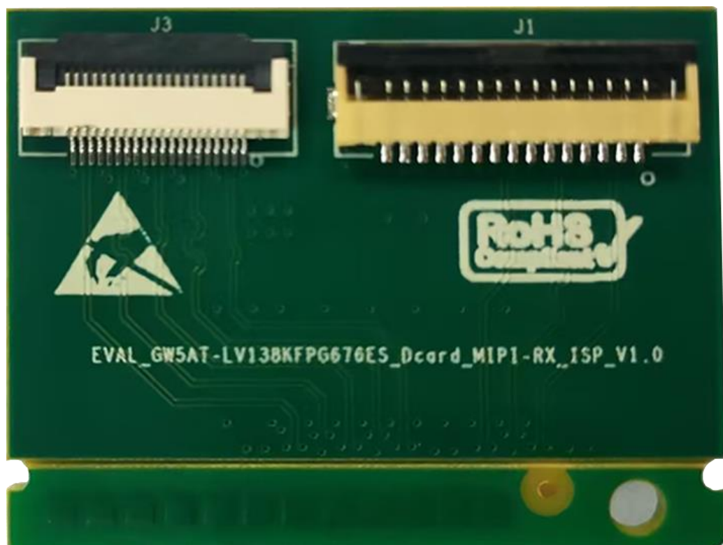
图 4-1 EVAL_GW5AT-LV138KFPG676ES_Dcard_MIPI-RX_ISP_V1.0 子板
