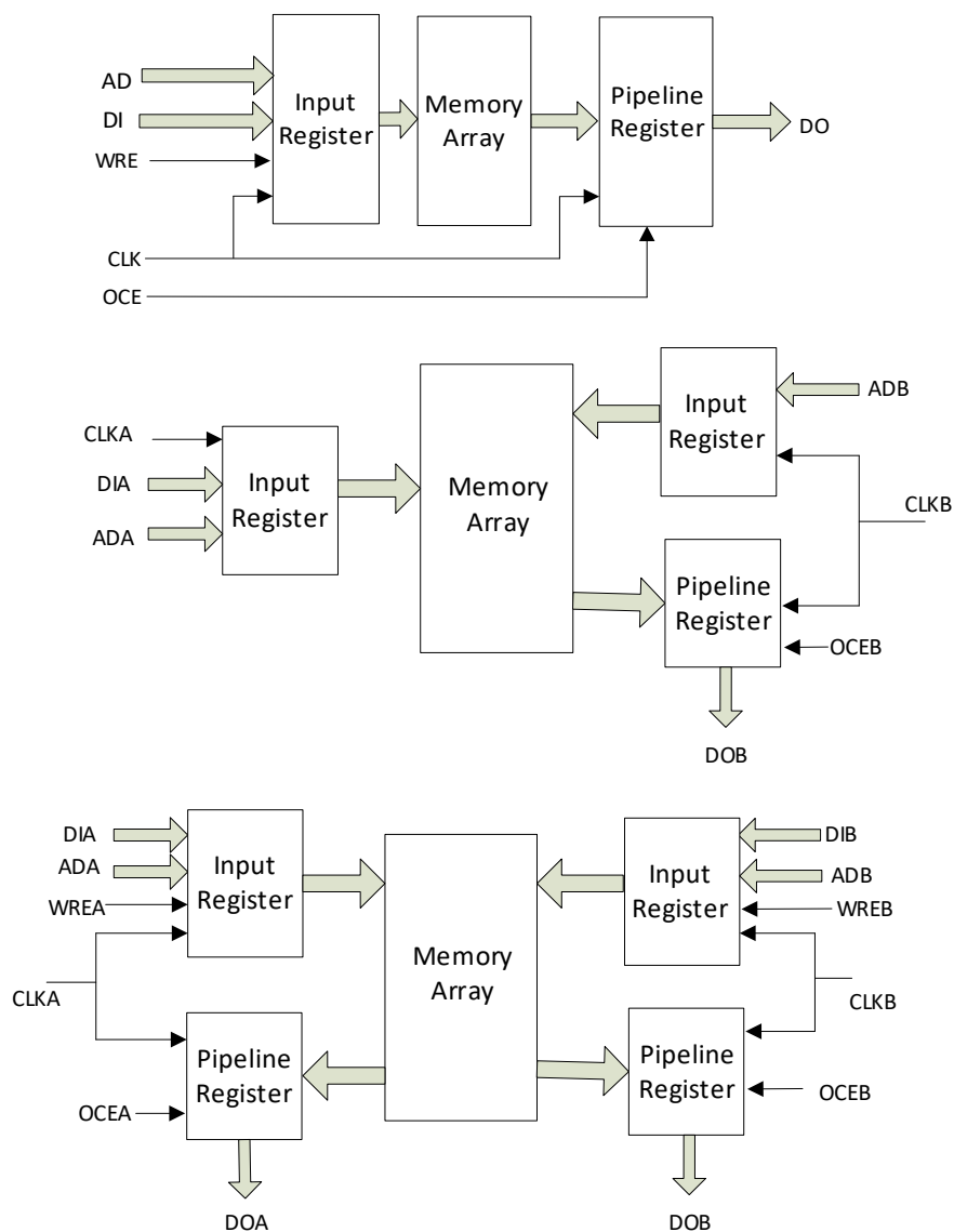
图 2-17 单端口、伪双端口及双端口模式下的流水线模式
