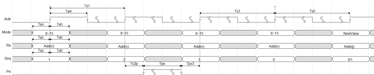
图 3-4 高电平周期
