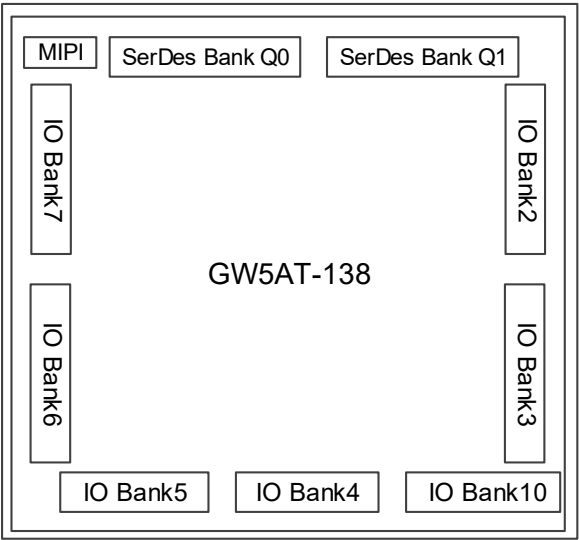
图 2-6 I/O Bank 分布示意图 (GW5AT-138)
