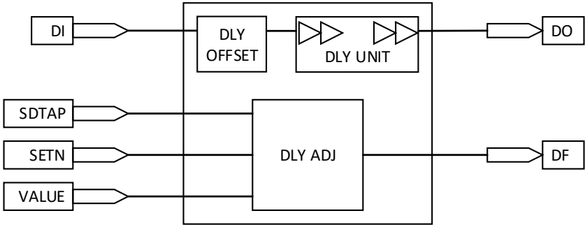
图 2-11 IODELAY 示意图
