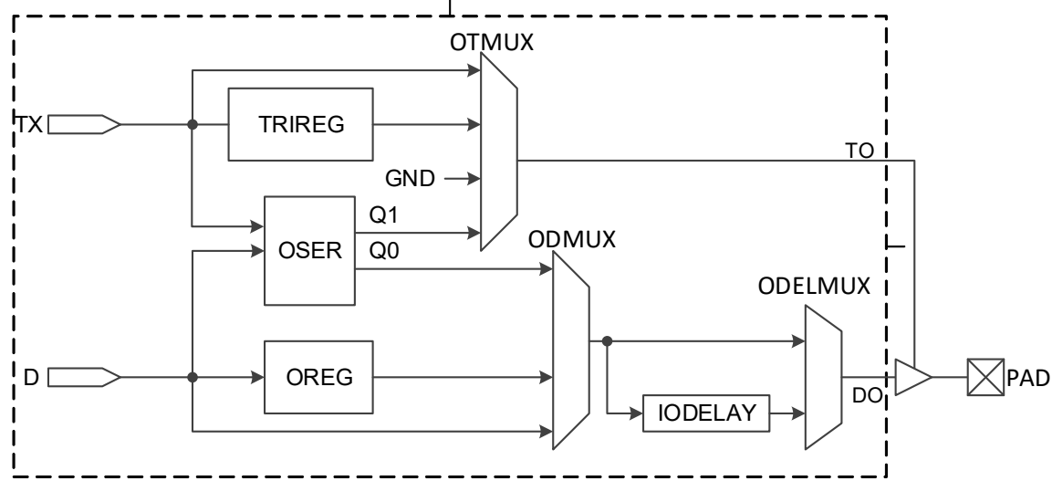
图 2-5 I/O 逻辑输出示意图
