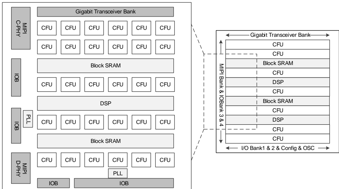
图 2-1 结构概念示意图 ( GW5AT-15)
