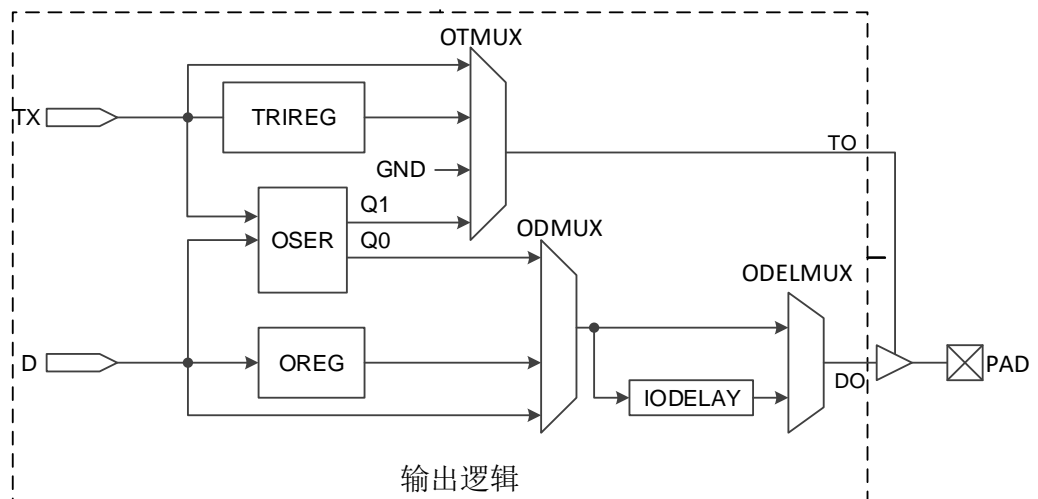
图 2-8 I/O 逻辑输出示意图
