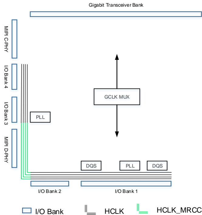
图 2-17 Arora V 15K FPGA 产品时钟资源
