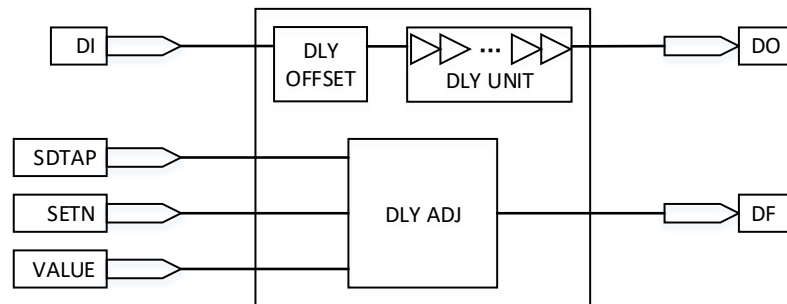
图 2-10 IODELAY 示意图
