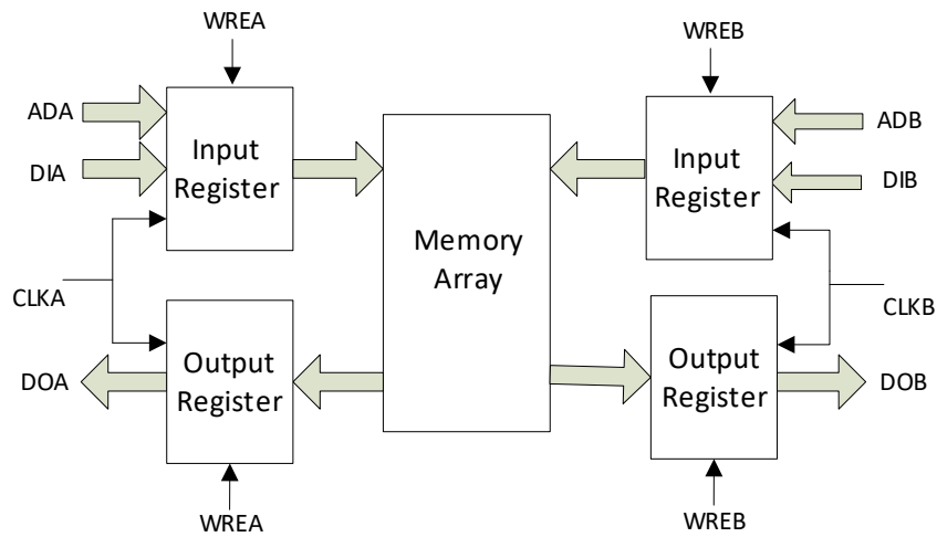
图 2-13 独立时钟模式
