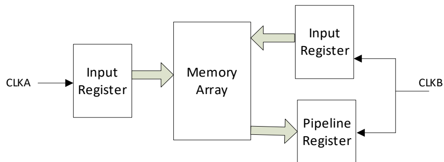
图 2-14 读写时钟模式
