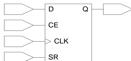
图 2-11 I/O 寄存器示意图
