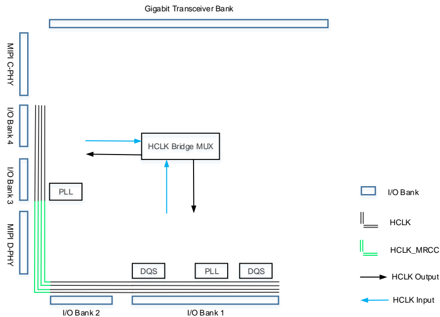
图 2-18 HCLK 示意图
