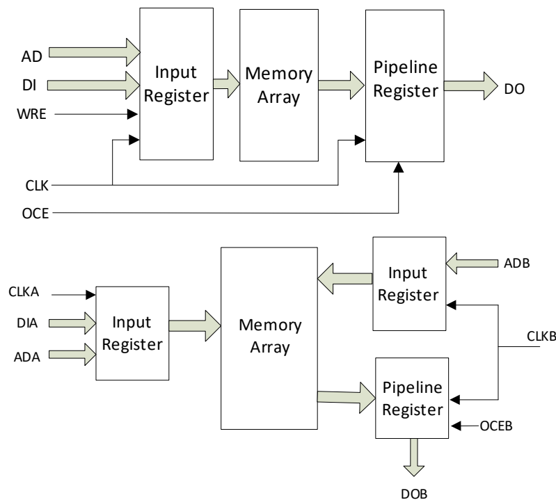
图 2-12 单端口、伪双端口及双端口模式下的流水线模式
