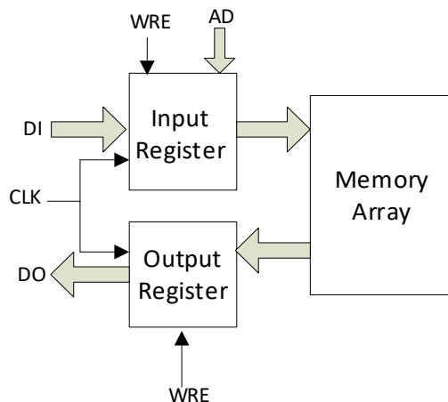
图 2-15 单端口时钟模式
