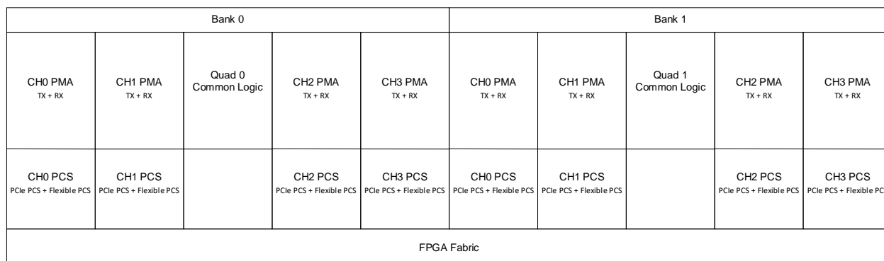
图 2-16 Gigabit Transceiver 结构示意图
