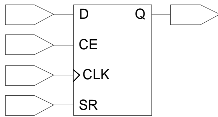
图 2-12 GW1NR 的 I/O 寄存器示意图
