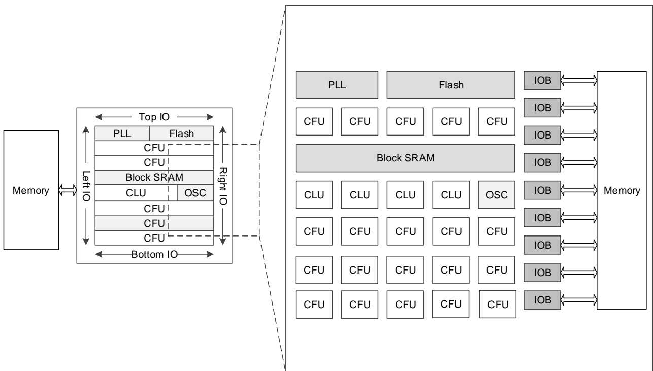
图 2-1 GW1NR-1 器件结构示意图
