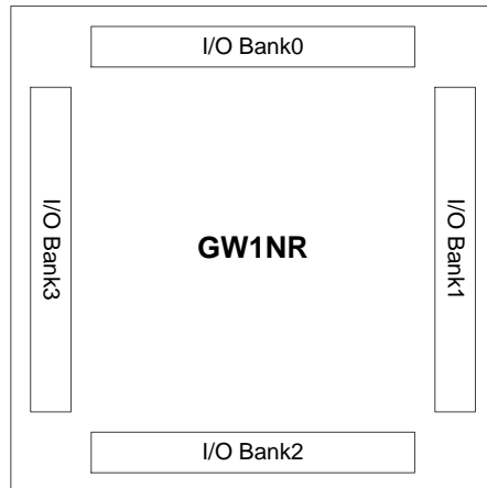
图 2-7 GW1NR-1/4/9 I/O Bank 分布示意图
