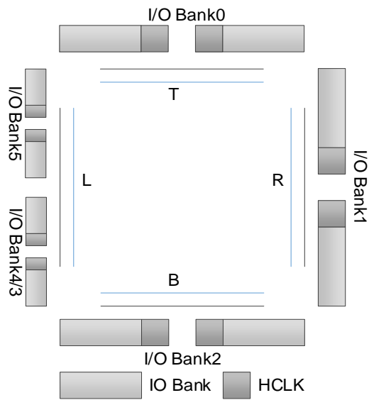
图 2-19 GW1NR-2 HCLK 示意图
