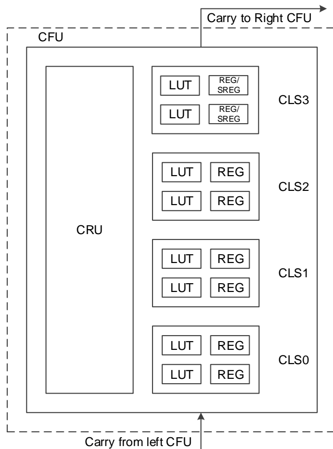
图 2-5 CFU 结构示意图
