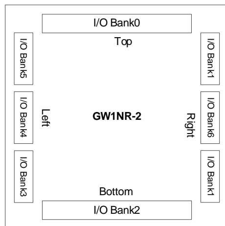
图 2-8 GW1NR-2 I/O Bank 分布示意图
