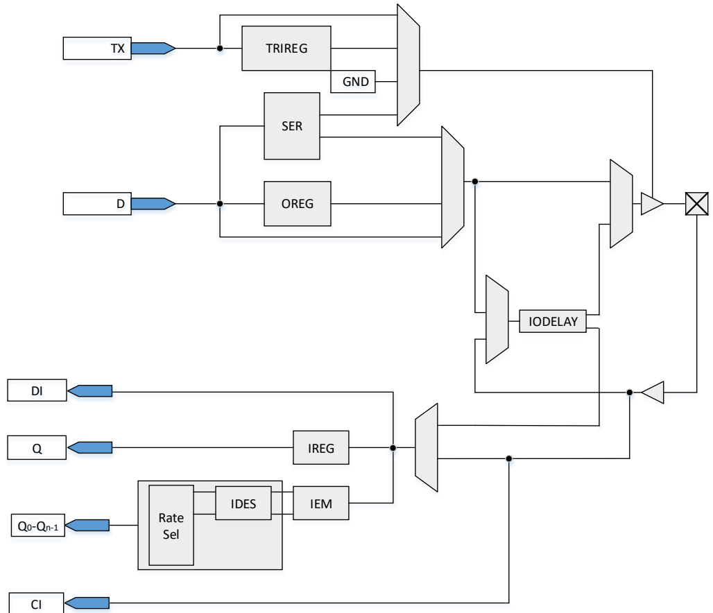
图 2-10 I/O 逻辑输入输出示意图
