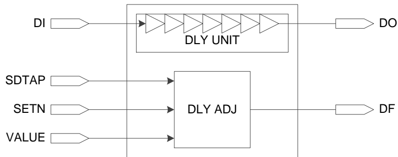
图 2-11 IODELAY 示意图
