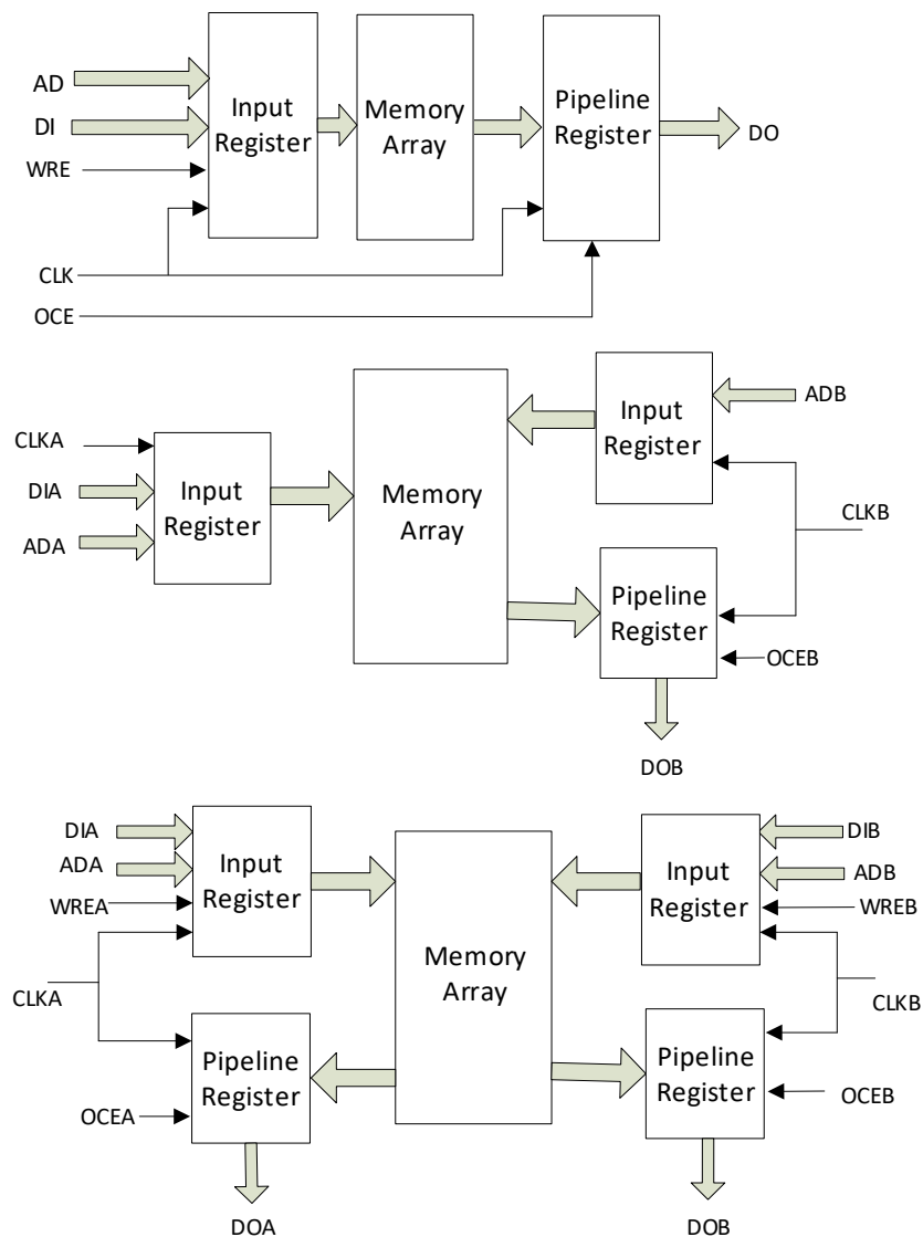
图 2-14 单端口、伪双端口及双端口模式下的流水线模式
