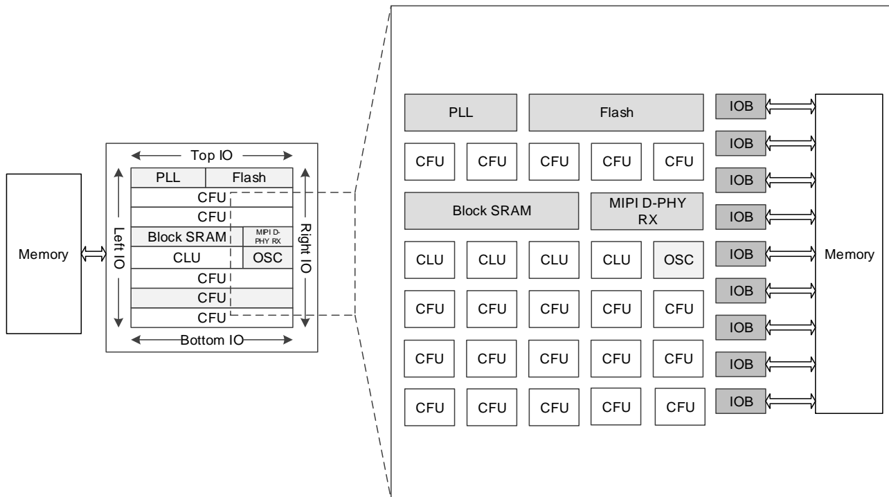
图 2-4 GW1NR-2 器件结构示意图
