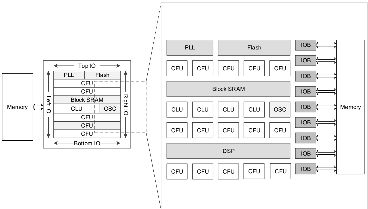
图 2-3 GW1NR-9 器件结构示意图
