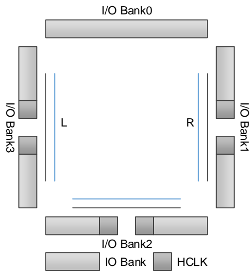
图 2-20 GW1NR-4 HCLK 示意图
