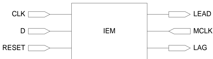
图 2-13 GW1NR 的 IEM 示意图
