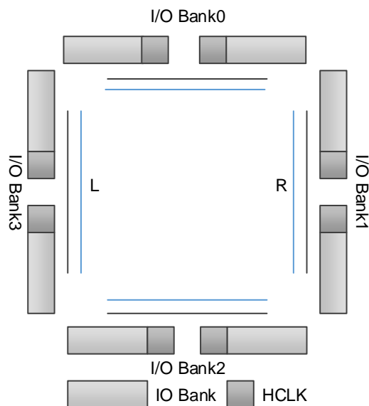
图 2-21 GW1NR-9 HCLK 示意图
