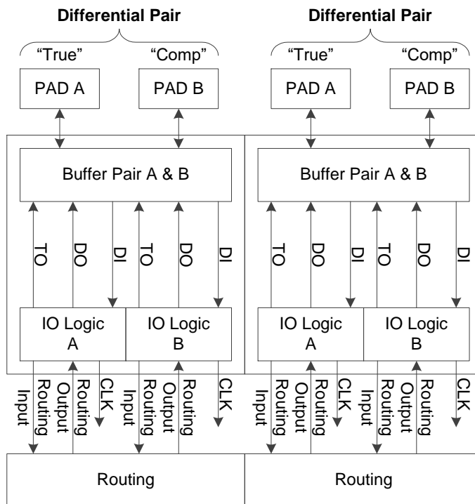
图 2-6 IOB 结构示意图
