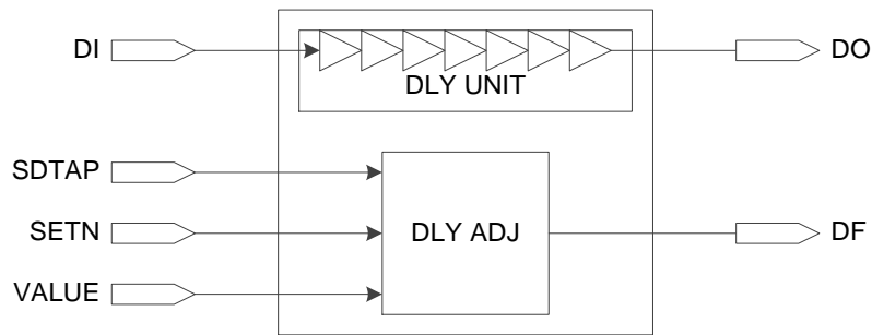
图 2-6 IODELAY 示意图
