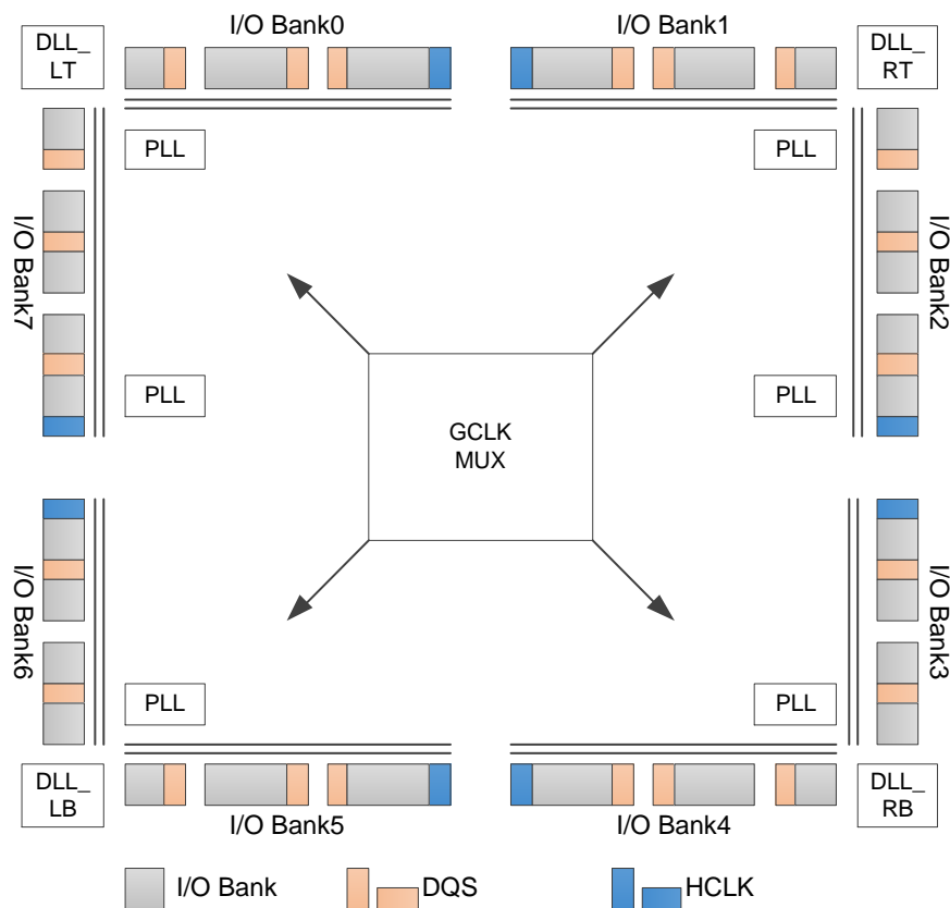
图 2-13 GW2AR 时钟资源
