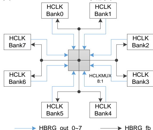
图 2-14 GW2AR HCLK 示意图
