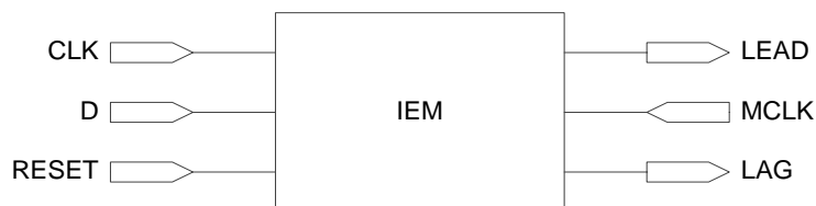
图 2-8 GW2AR 的 IEM 示意图
