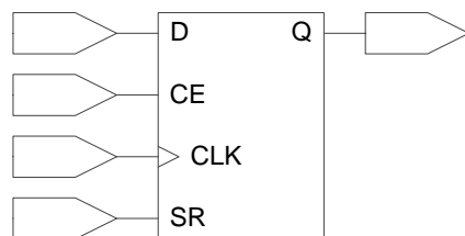
图 2-7 GW2AR 的 I/O 寄存器示意图
