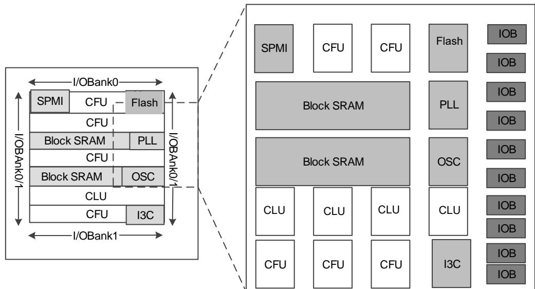
图 2-2 GW1NZ-2 器件结构概念示意图
