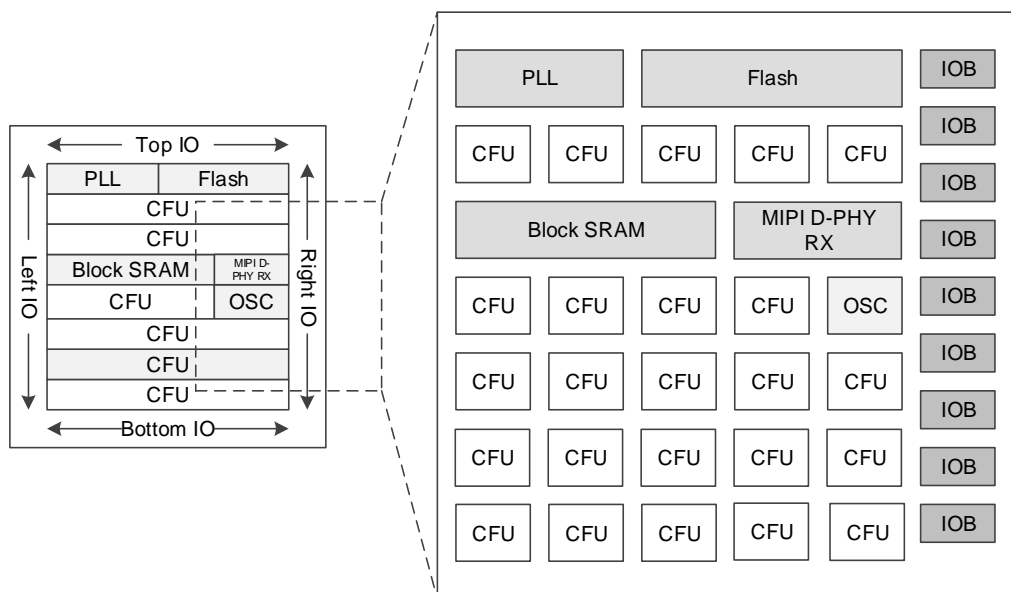
图 2-2 GW1NZ-2 器件结构概念示意图
