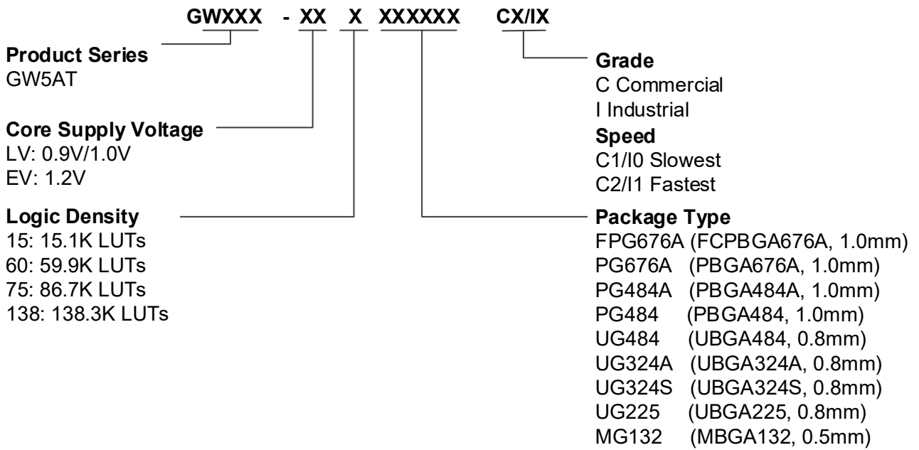
图 4-2 器件命名方法示例-Production
