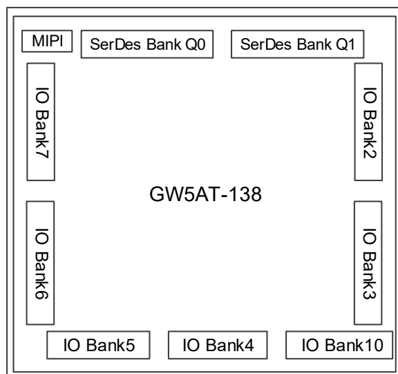
图 2-7 I/O Bank 分布示意图 (GW5AT-138)
