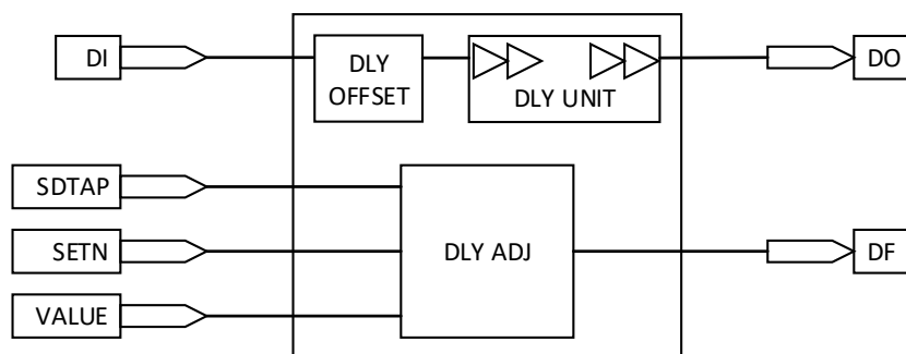
图 2-13 IODELAY 示意图
