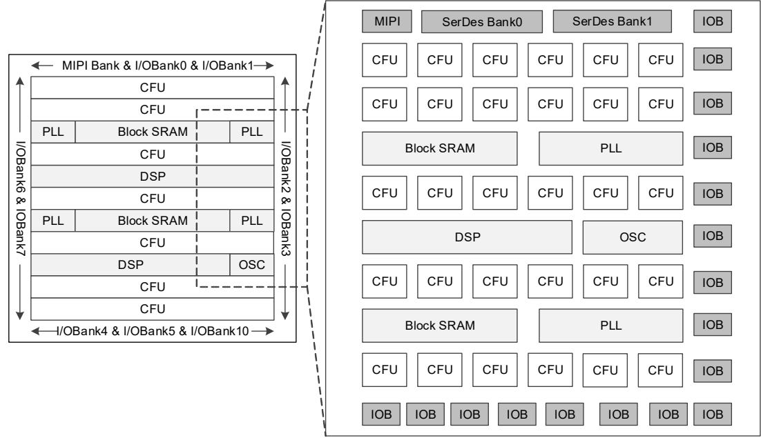
图 2-3 结构概念示意图（GW5AT-60）
