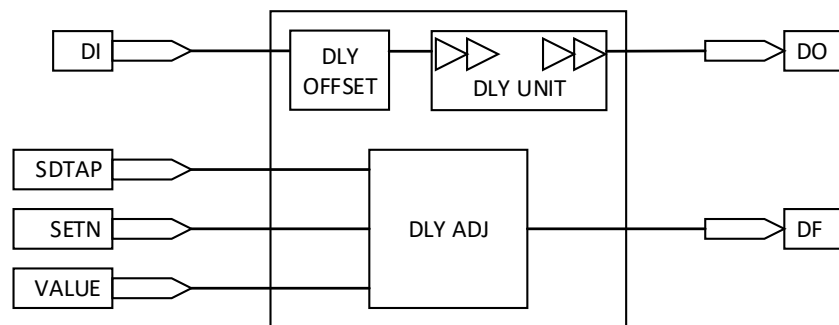
图 2-13 IODELAY 示意图
