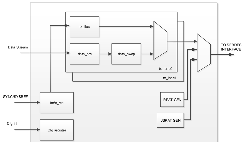
图 3-1 发送器结构图
