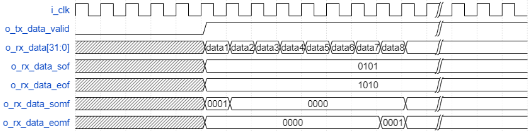
图 3-9 F=2 K=32 时，接收数据接口时序
