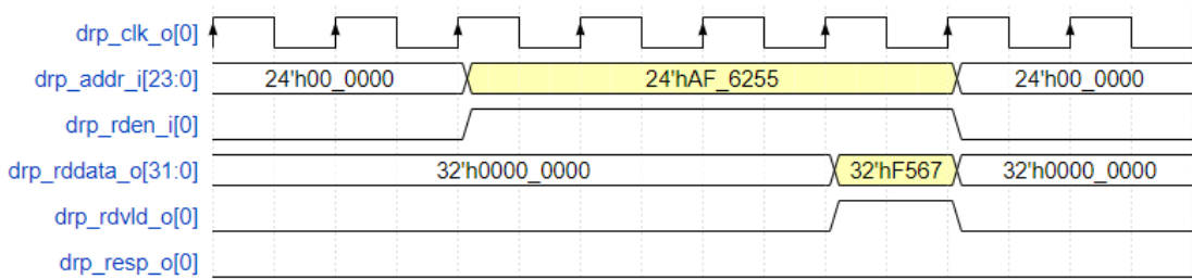
图 3-10 DRP 接口读时序图
