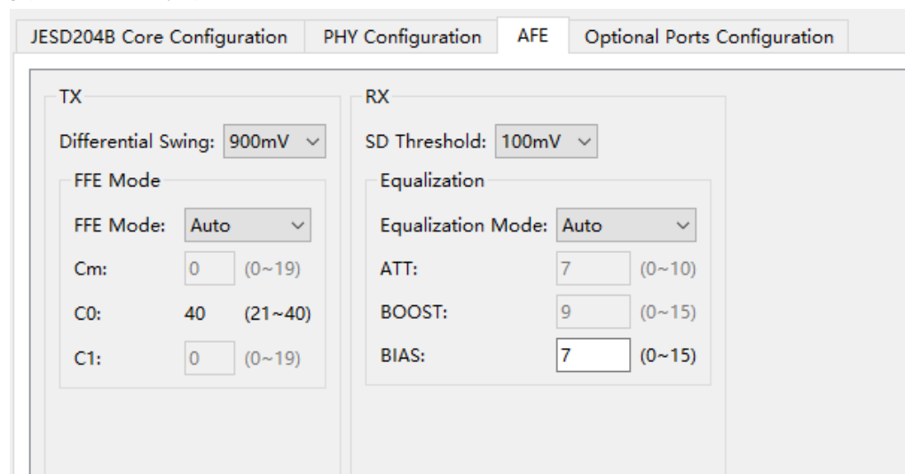
图 5-4 AFE 选项卡
