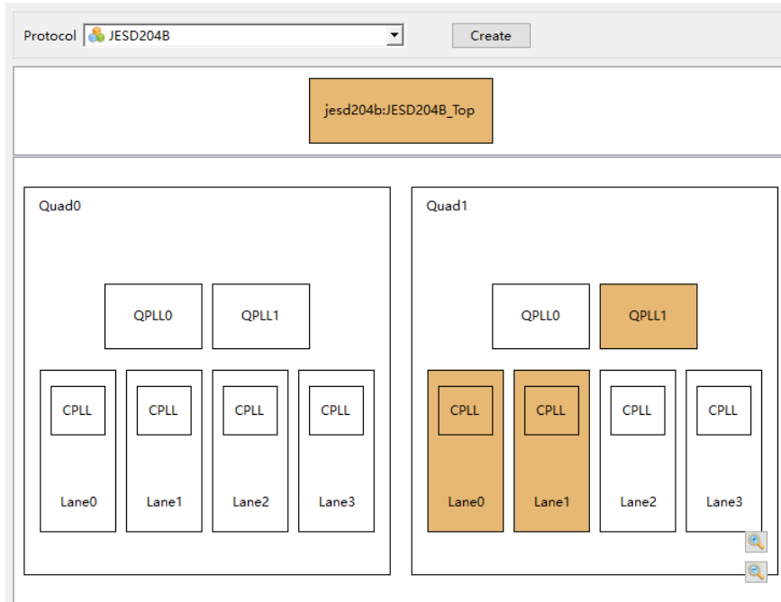
图 5-6 jesd204b: JESD204B_Top
