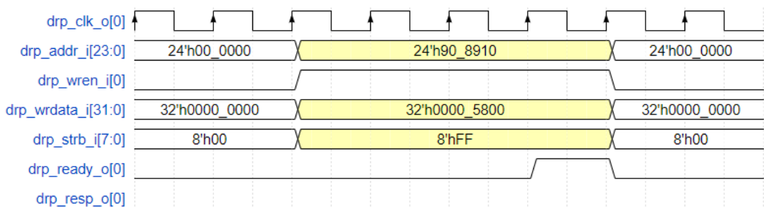
图 3-11 DRP 接口写时序图
