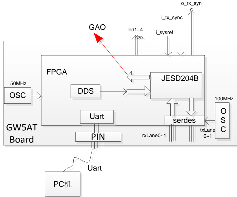
图 6-3 平台框图
