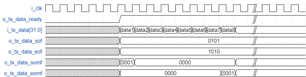
图 3-8 F=2 K=32 时，发射数据接口时序
